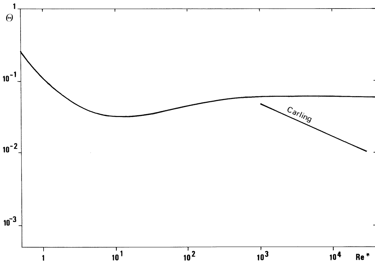
Figure 5 : Variation du critère de Shields \theta en fonction de Re^* (d'après Graf, 1971) et relation trouvée en rivière naturelle par Carling (1983) dans l'Eggeshape Beek.
