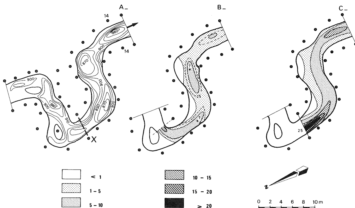
Figure 7 : Répartition des forces tractrices dans un secteur de la Rulles, en B pour le débit moyen, en C pour un débit proche du débit à pleins bords (en N.m^{-2} ). En A, morphologie du secteur: équidistance des courbes de niveau de 10 cm, élévation par rapport à un niveau de référence arbitraire.
