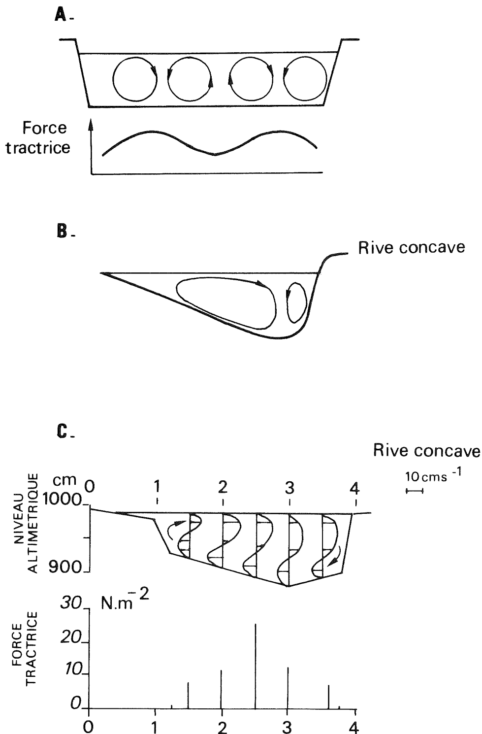
Figure 6 : A. Schéma de l'organisation de la circulation secondaire en un système multicellulaire, propre aux rivières subrectilignes peu profondes et effet sur la force tractrice s'exerçant sur le lit (d'après Bathurst et al. , 1979 et Richards, 1982)
