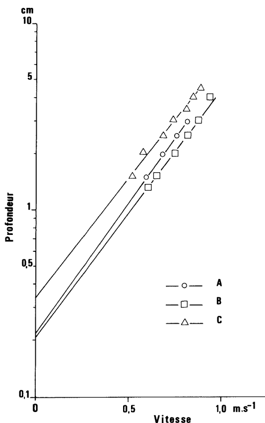
Figure 1 : Détermination du paramètre de rugosité y_0 , par application de la loi de la paroi : A et B, exemples pris en flume à fond caillouteux ( D_{90} = 1,96 cm) pour les essais effectués avec un débit de 56 \text{ l.s}^{-1} et de 95 \text{ l.s}^{-1} ( y_0 = 0,22 cm et y_0 = 0,21 cm respectivement). C, exemple pris dans la Burdinale avec un D_{90} = 6,02 cm ( y_0 = 0,35 cm).
