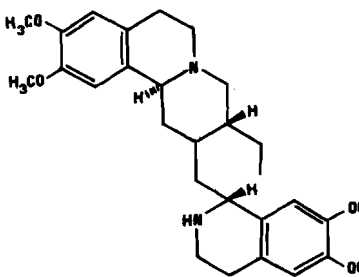
EMETINE
