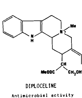
FIG. 10. Diploceline.
