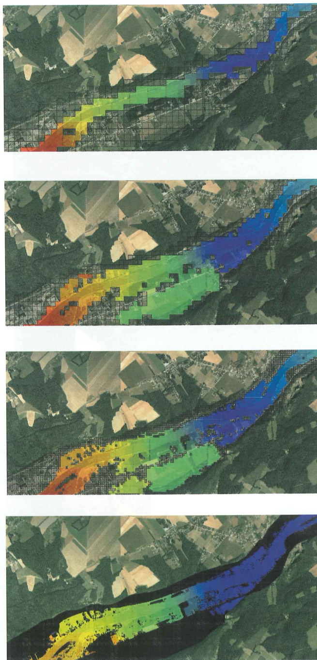
Figure 18 – Quatre maillages successifs illustrant le raffinement automatique mis en œuvre pour la détermination des zones inondées à Bas-Oha sur la Meuse, lors de la crue de 1995.
