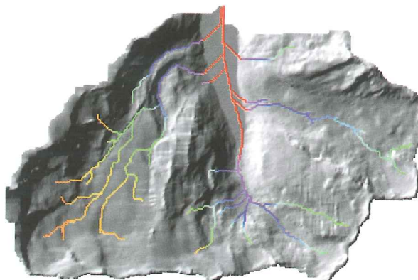
Figure 7 – Bassin versant et réseau drainant automatiquement généré par WOLF HYDRO.
