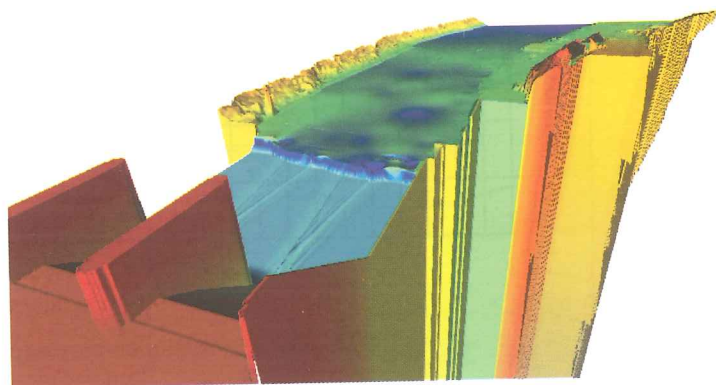
Figure 15 – Résultat de la simulation numérique de l'ouvrage.
