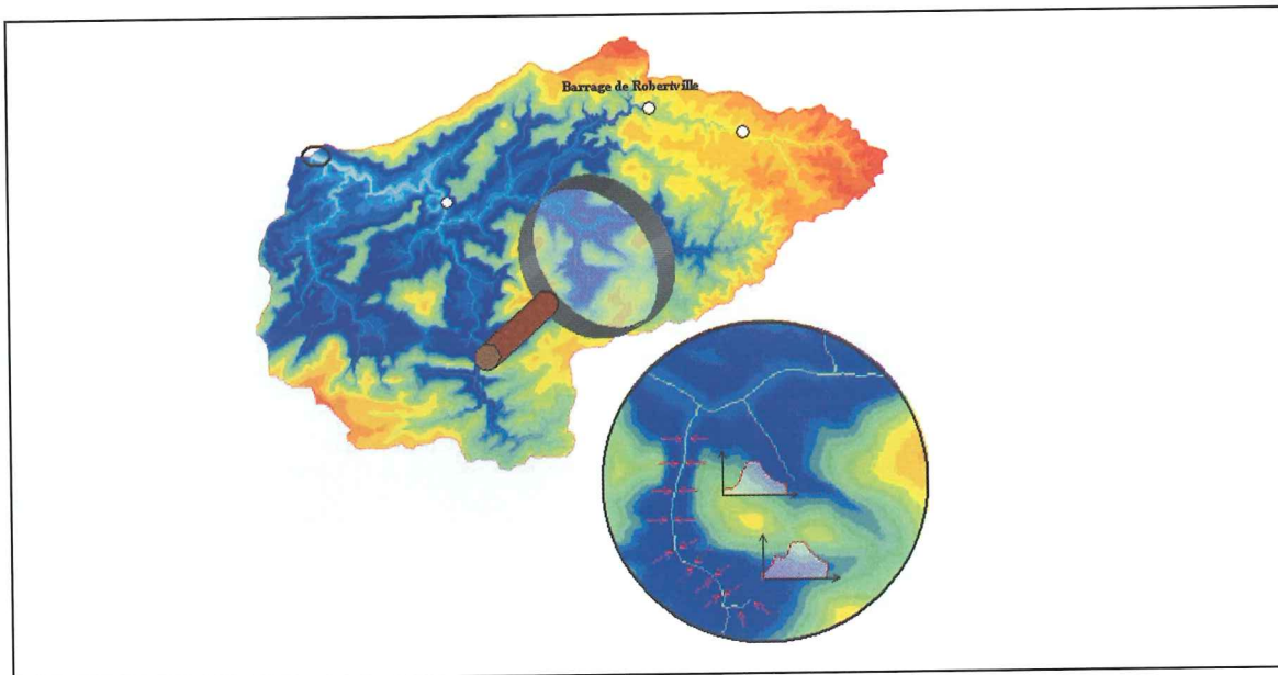
Figure 9 – Topographie du bassin de l'Amblève (Belgique) et schéma du mécanisme d'apports latéraux dans le réseau de rivières.
