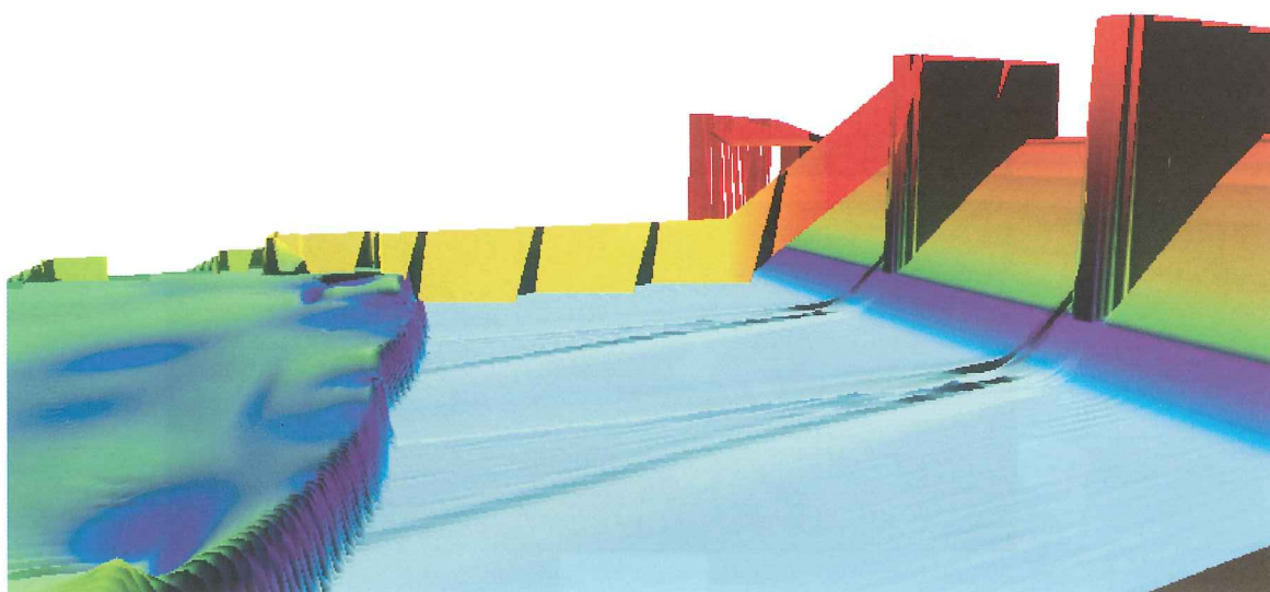
Figure 17 – Vue tridimensionnelle de l'écoulement sur le coursier et dans le bassin de dissipation pour une crue de 175 m³/s.
