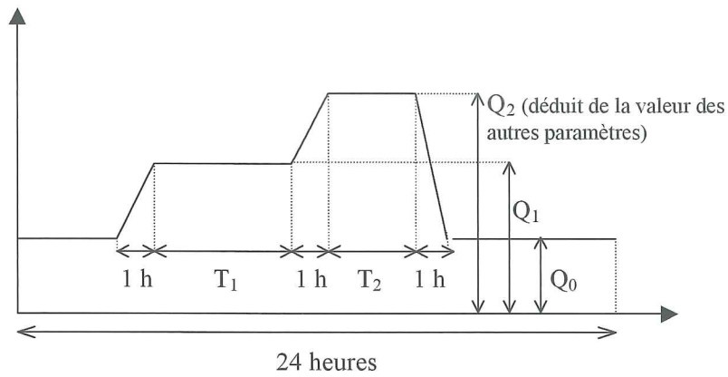
Figure 11 – Hydrogramme paramétré.
