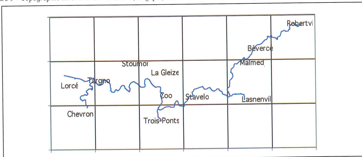
Figure 10 – Réseau de rivière modélisé.
