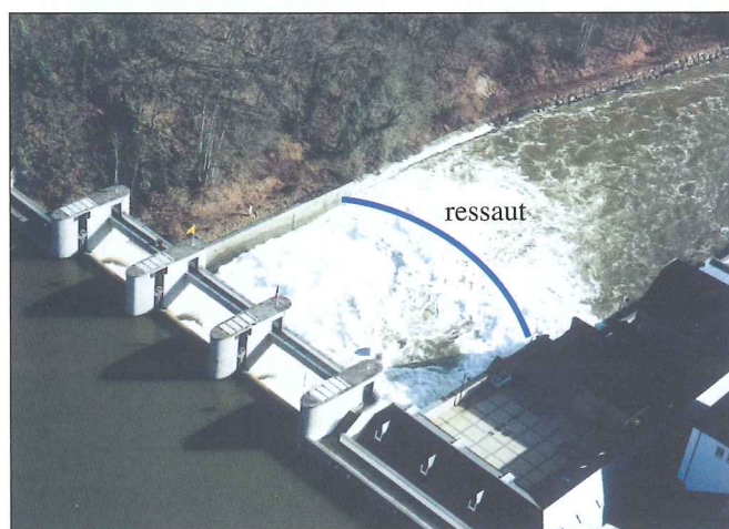
Figure 16 – Vue 3D du barrage, de la fosse de dissipation et de l'écoulement sur la structure.
