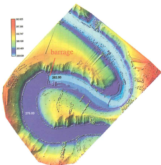
Figure 14 – Topographie complète du site étudié.
