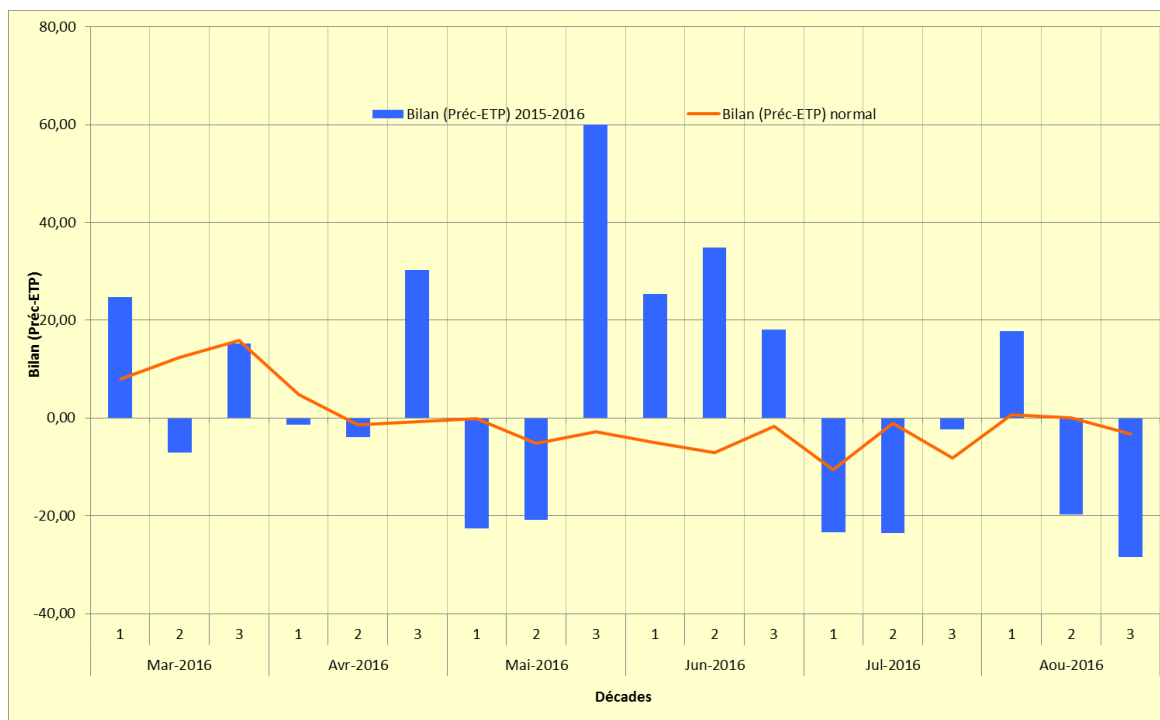
Figure 1.7 : Bilan (Précipitations – ETP) 2015-2016 et bilan (Précipitations – ETP) normal en mm, par décennie du 1 er mars 2016 au 31 août 2016 au poste climatologique d'Ernage-Gembloux (IRM).
