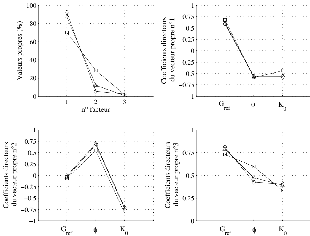
FIG. 4.51 – Pressiomètre synthétique : Identification des paramètres de Mohr-Coulomb G_{ref} , \phi et K_0 . Valeurs propres et vecteurs propres des matrices de corrélations déduites de trois optimisations avec N_{individus} = 540 individus.
