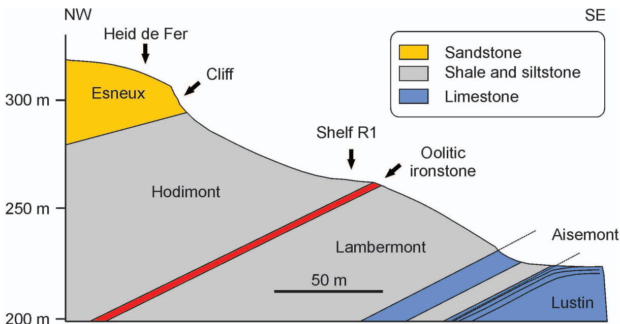
Fig 4 – Schematic cross section of the Heid de Fer site. Coupe schématique à travers du site de la Heid de Fer.
