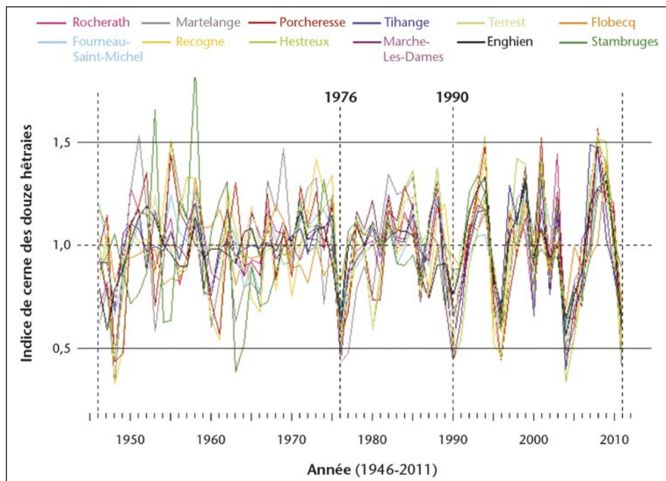
Figure 1 – Synchronisation progressive de la variation annuelle de l'accroissement des douze hêtraies, réparties le long du gradient altitudinal de Wallonie, en réponse à l'influence grandissante du changement climatique. Trois périodes peuvent être distinguées : avant 1976 (signal commun faible), entre 1976 et 1990 (début de synchronisation) et après 1990 (synchronisation très importante).
