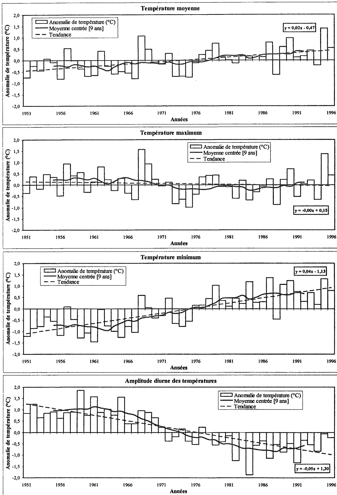
Fig.VI.8 - Evolution régionale en saison sèche (octobre à avril) des températures moyennes, maximales, minimales et des amplitudes thermiques diurnes moyennes durant la période 1951-1996. Ecarts de températures calculés par rapport à la moyenne 1961-1990 suivant l'équation III. 2.
