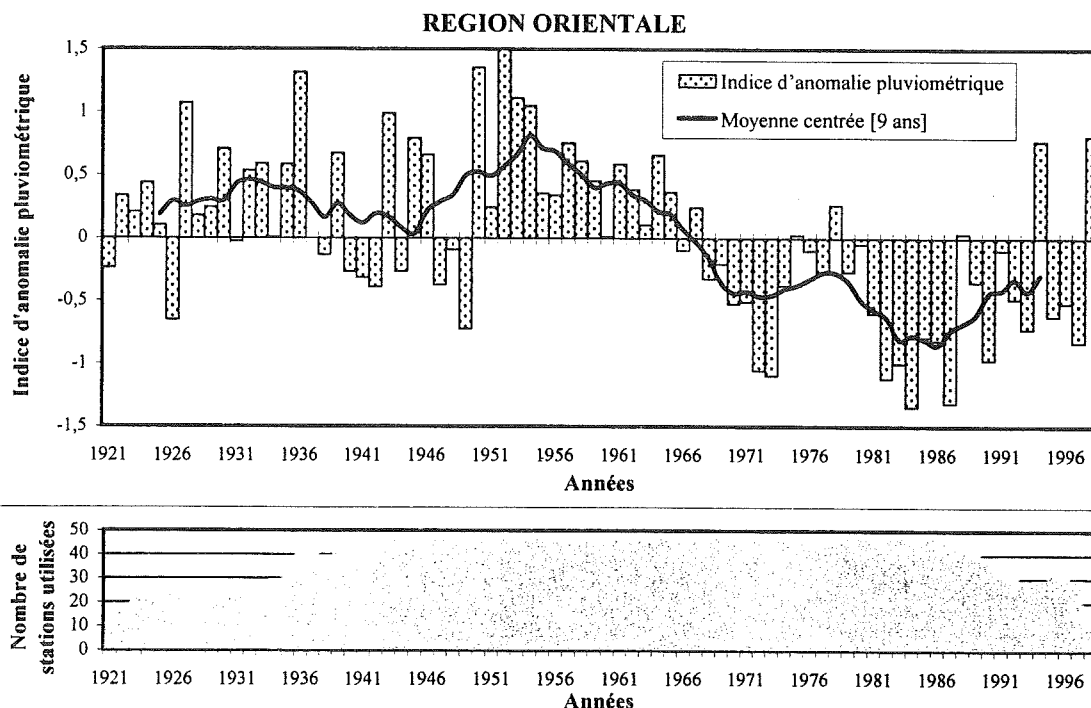
Fig.III.4 - Evolution régionale (Mali et Niger) des précipitations de 1921 à 1998 exprimée en fonction de l'indice d'anomalie pluviométrique" (LAMB 1982). Le nombre de stations prises en compte pour le calcul de l'indice d'anomalie pluviométrique" est présenté dans le graphique inférieur.
