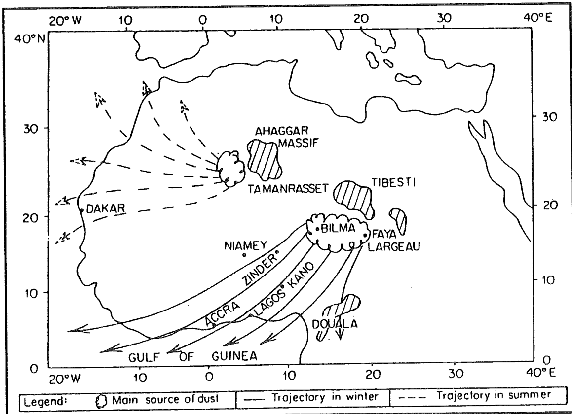
Fig.IV.52 - Zones sources principales de poussières décrites par KALU (1979).
