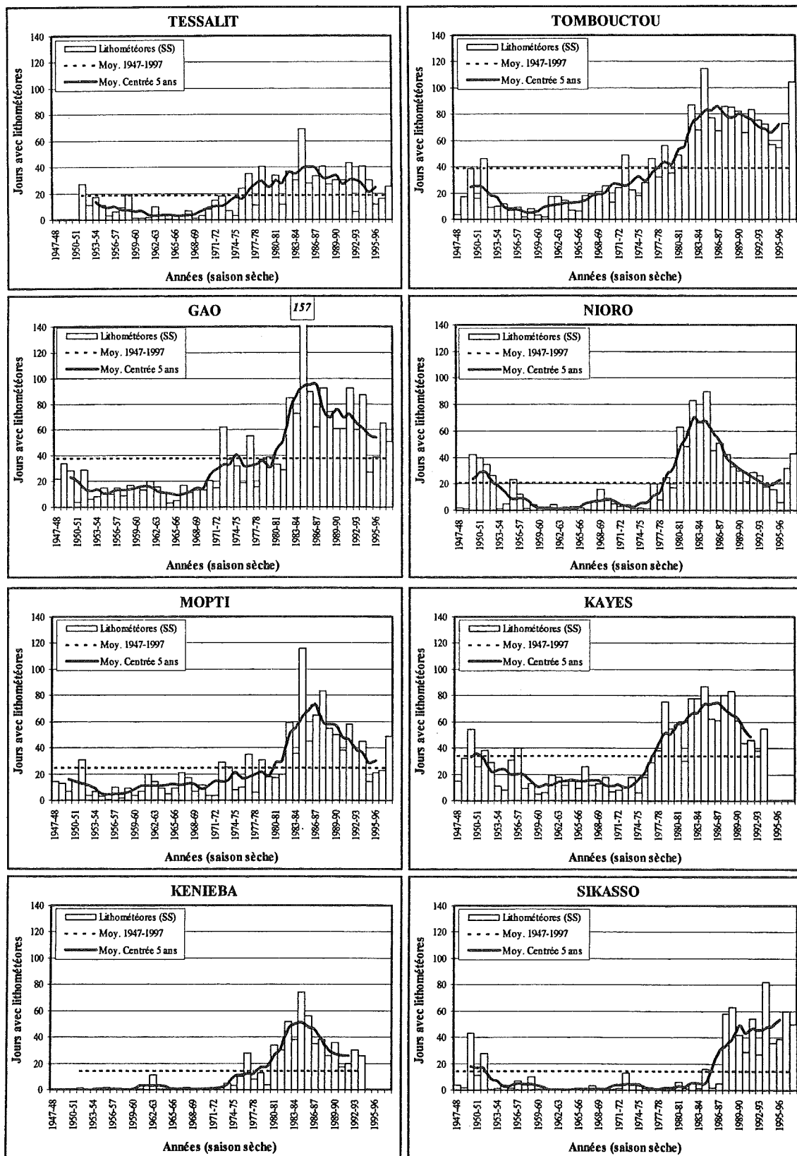
Fig.IV.35 - Evolution du nombre de jours affectés par les lithométéores en saison sèche (octobre – avril) au Mali de 1947-48 à 1997-98. La moyenne détermine la période utilisée pour chaque station.
