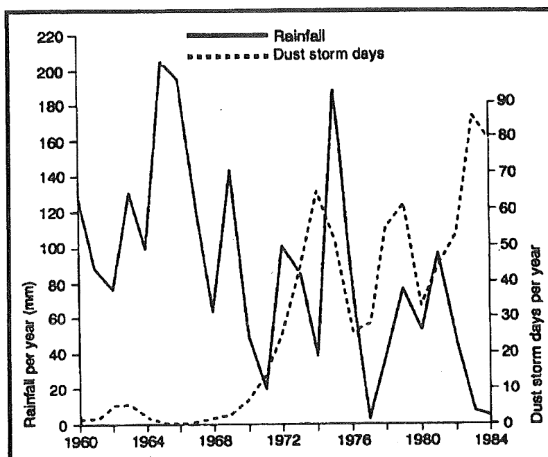
Fig.IV.13. - Fréquences annuelles des tempêtes de sable 1 et totaux annuels des précipitations à la station de Nouakchott de 1960 à 1984 (d'après MIDDLETON 1985A)
