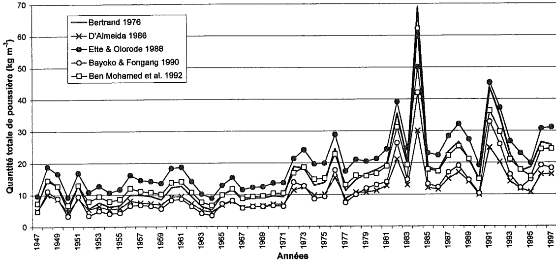
Fig.IV.65 - Evolution, de 1947 à 1997, de la quantité totale de particules solides ( \text{kg m}^{-3} ) ayant transité par une surface verticale de 1 \text{ m}^2 à une hauteur de dix mètres au-dessus du sol durant la saison sèche courte (novembre à mars) à la station de Niamey. Toutes les visibilitées tri-horaires sont prises en compte. Les concentrations en poussières sont dérivées des équations IV. 7, 11, 13, 14 et 15 présentées au tableau IV. 29. Moyenne 1947-1997: BERTRAND (1976): 16.3; D'ALMEIDA (1986): 10.7; ETTE et OLORODE (1988): 20.3; BAYOKO et FONGANG (1990): 11.8; BEN MOHAMED et al. (1992): 15.8.
