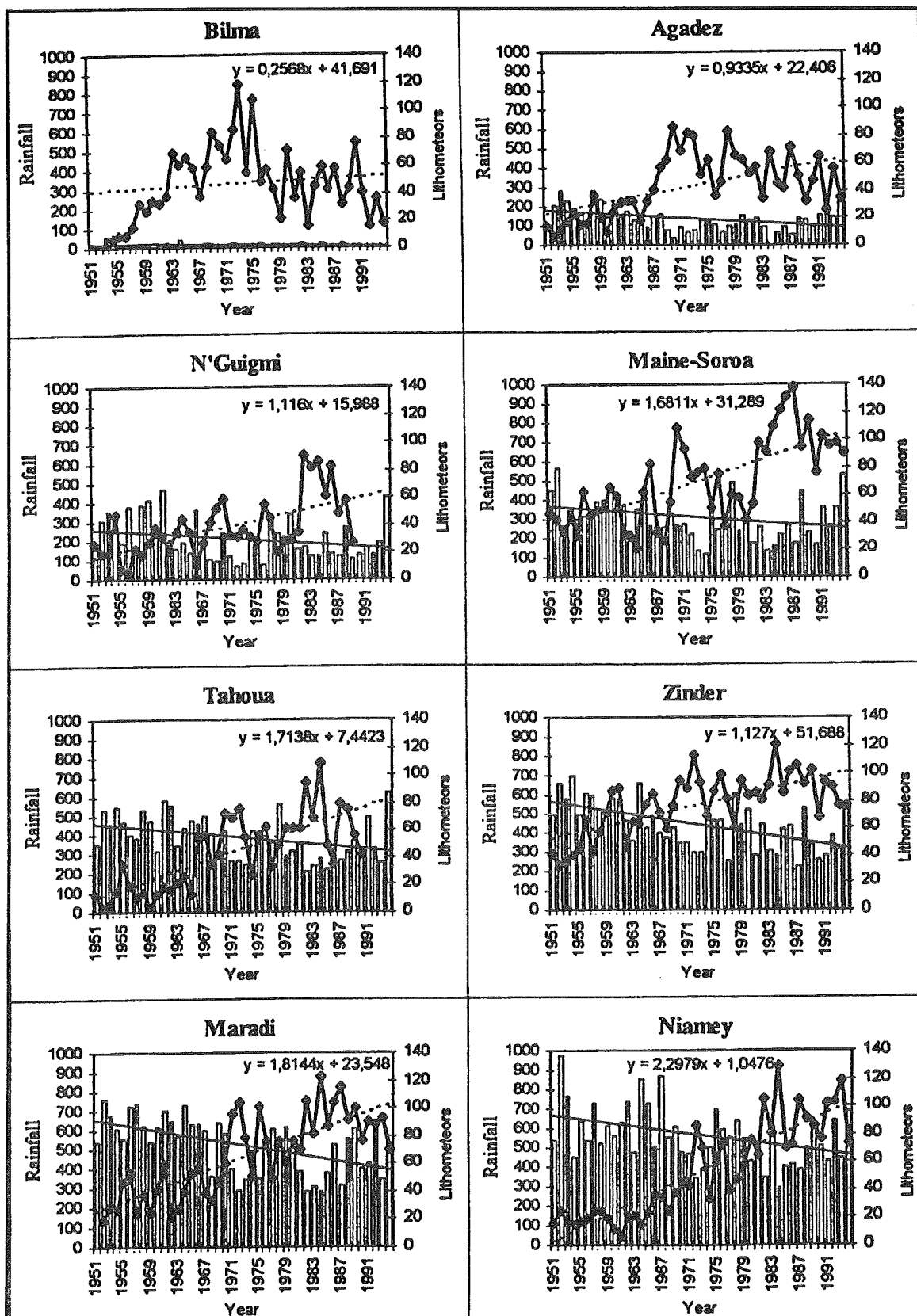
Fig.IV.16 - Evolution des précipitations annuelles (bâtons) et du nombre de jours affectés par les lithométéores (courbe); durant la saison sèche de 1951 à 1994 dans huit stations synoptiques du Niger (OZER 1998).
