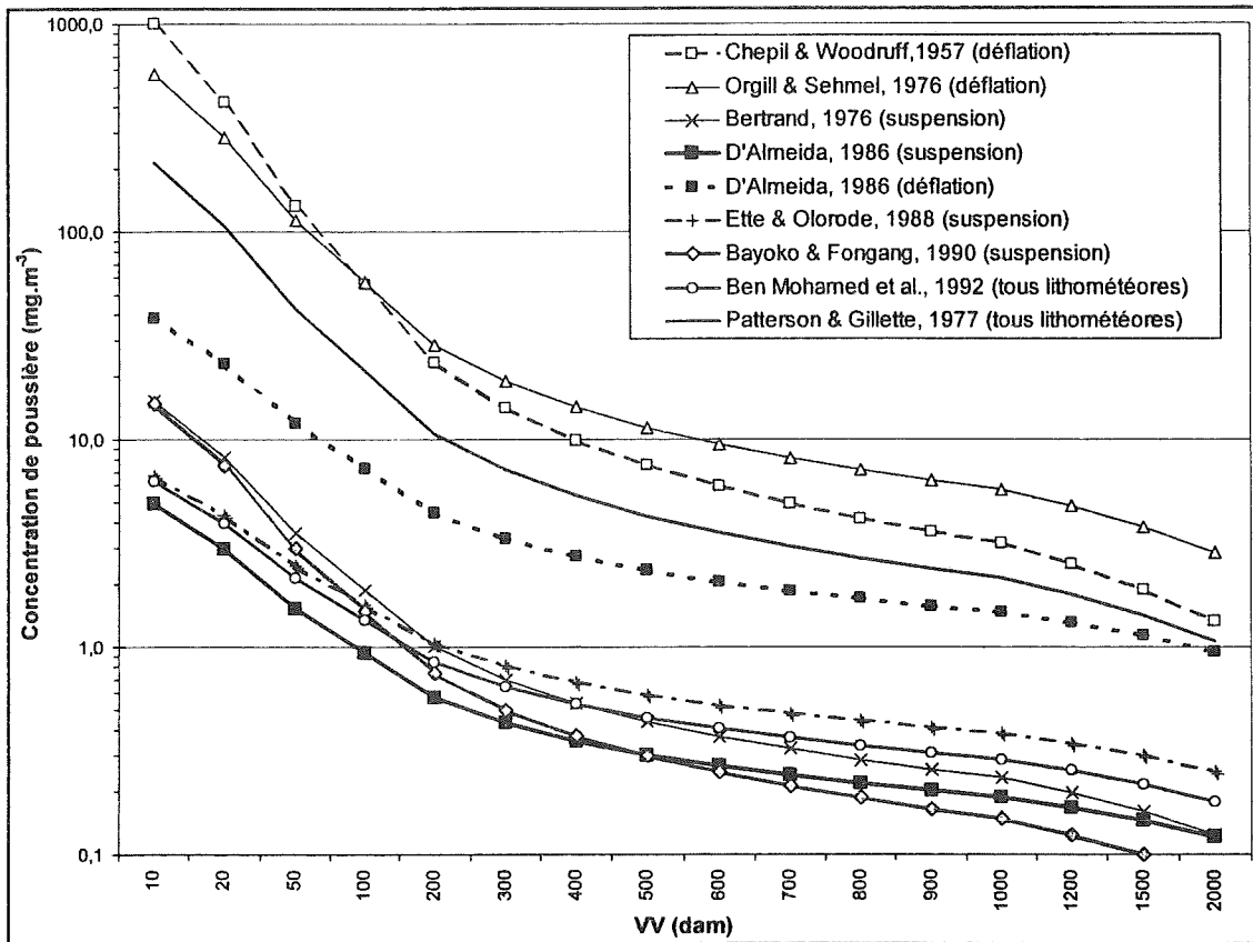
Fig.IV.63 - Relation entre visibilité et concentration en particules solides (déflation et suspension) dans l'atmosphère suivant divers auteurs.
