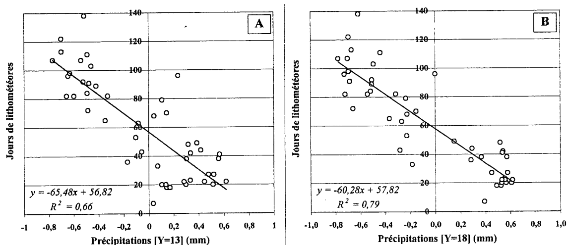
Fig.IV.58 - Relation maximum entre la fréquence des lithométéores à Niamey et [A] la pluviométrie moyenne locale (Y=13) et [B] la pluviométrie moyenne régionale (Y=18). Les précipitations sont traduites en valeurs centrées réduites suivant la méthode de LAMB (1982).
