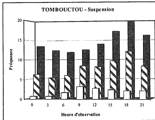
Fig.IV.25 - Fréquence moyenne (%) tri-horaire de la visibilité réduite par les poussières en suspension et les cas de déflation durant la saison sèche (novembre à mars) aux stations de Gao et Tombouctou. Comparaison entre les périodes "humide" (1951-1968, blanc), de sécheresse (1969-1986, hachuré), et "actuelle" (1987-1997, noir).
