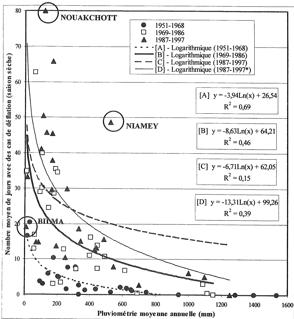
Fig.IV.53 - Fréquence des cas de déflation (jours par saison sèche), en relation avec les précipitations moyennes (mm) durant les périodes "humide" (1951-1968), de sécheresse (1969-1986) et "actuelle" (1987-1997). * Equation logarithmique ajustée aux valeurs obtenues pour la période 1987-1997 sans les stations de Niamey et Bilma.
