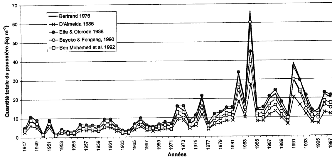
Fig.IV.66 - Cf. Fig. IV.65 uniquement pour les visibilitées tri-horaires inférieures à 1000 dam. Moyenne 1947-1997: BERTRAND (1976): 12.3; D'ALMEIDA (1986): 6.9; ETTE et OLORODE (1988): 12.7; BAYOKO et FONGANG (1990): 9.3; BEN MOHAMED et al. (1992): 10.2.
