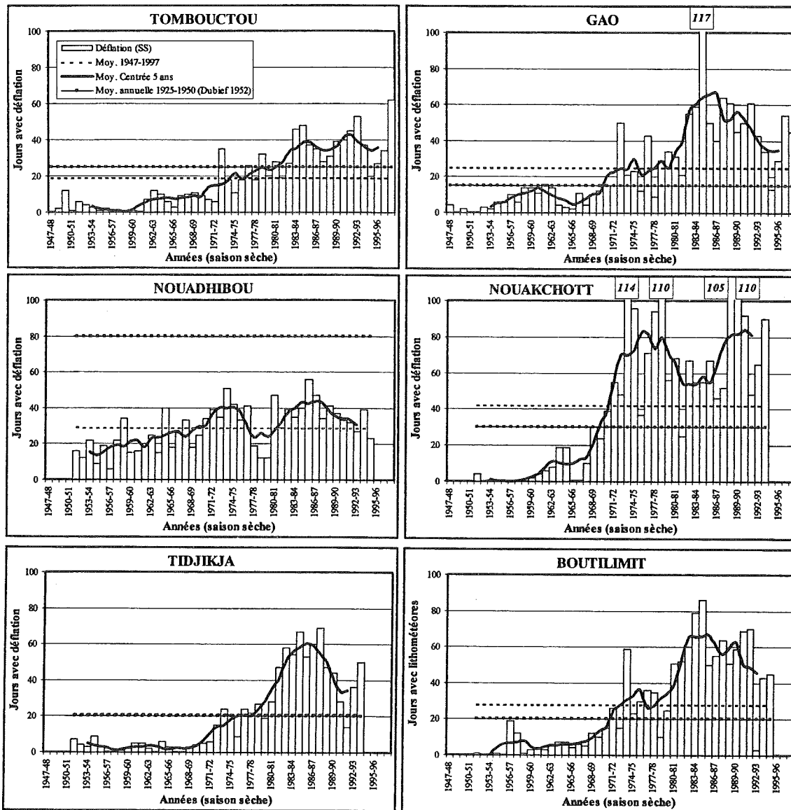
Fig.IV.44 - Evolution des cas de déflation en saison sèche (octobre - avril ) au Mali et en Mauritanie de 1947-48 à 1997-98. La ligne moyenne (pointillés) détermine la période utilisée pour chaque station. Comparaison avec les moyennes annuelles calculées par DUBIEF (1952) pour la période 1925-1950
