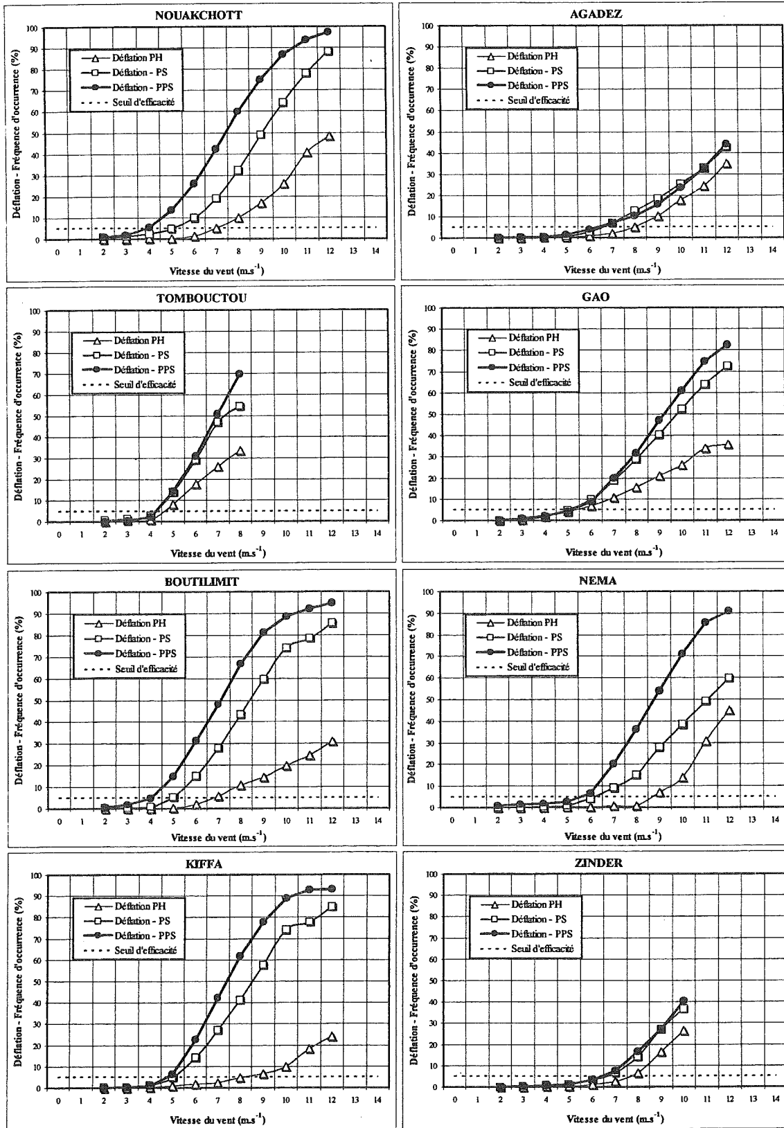
Fig.V.25 - Evolution de la fréquence d'observation des jours avec déflation en fonction de la vitesse du vent ( m s^{-1} ) dans huit stations de la zone d'étude. Comparaison entre les périodes "humide" (PH: 1951-1968), de sécheresse (PS: 1969-1986) et "actuelle" (PPS: 1987-1997).
