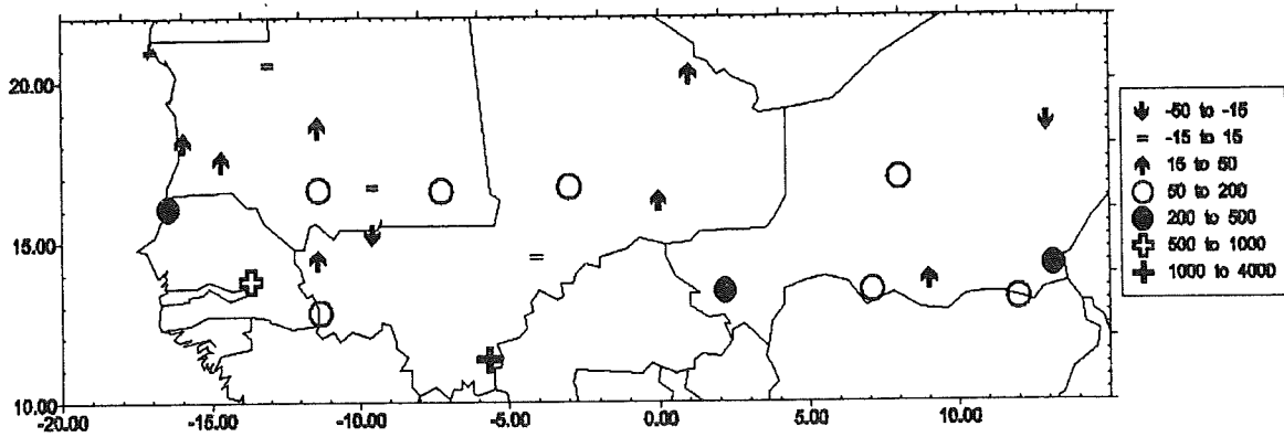
Fig.IV.48 - Evolution de l'occurrence des cas de déflations entre les périodes "actuelle" (1987-1997) et de sécheresse (1969-1986). La légende présente l'évolution (en %) entre ces deux périodes. Evolution of the deflation frequency between the "present" (1987-1997) and the drought (1969-1986) periods. The legend shows the evolution (%) between these two periods.
