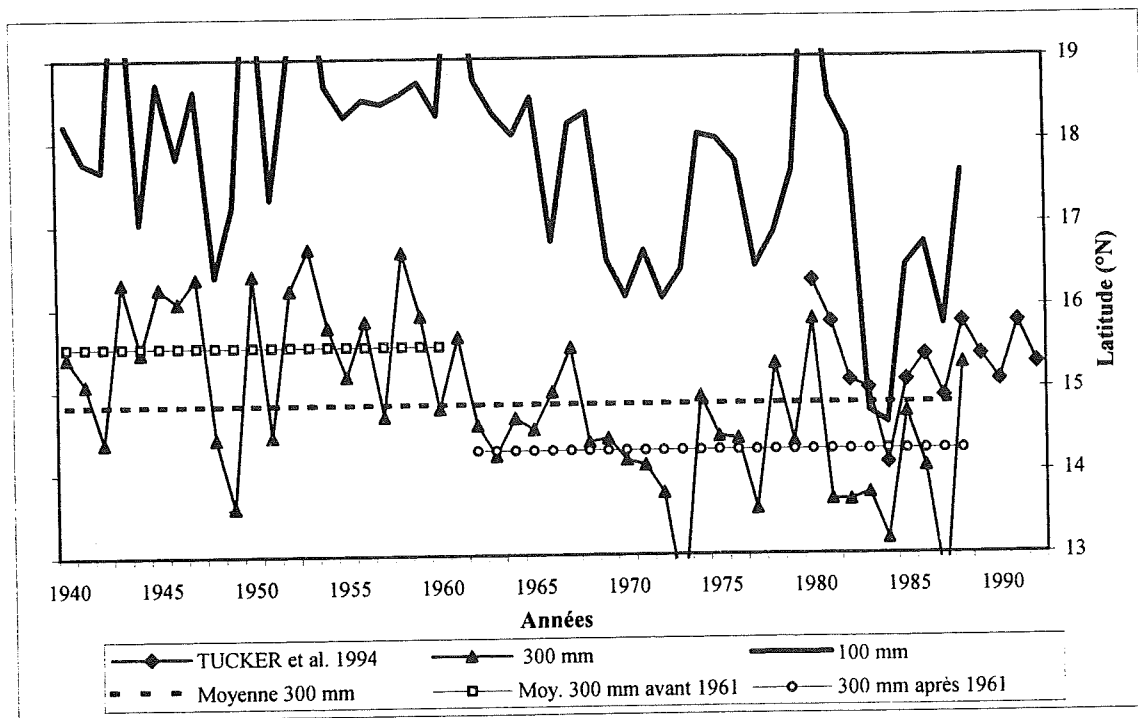
Fig.III.11 - Transect pluviométrique spatio-temporel de 13 à 18°N au centre du Niger (extrait de la Fig.III.10) et comparaison avec les données de TUCKER et al. (1994).
