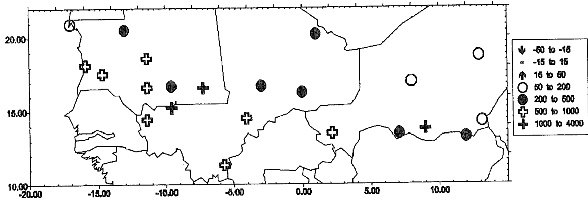
Fig.IV.47 - Evolution de l'occurrence des cas de déflation entre les périodes de sécheresse (1969-1986) et "humide" (1951-1968). La légende présente l'évolution (en %) entre ces deux périodes Evolution of the deflation frequency between the drought (1969-1986) and the "humid" (1951-1968) periods. The legend shows the evolution (%) between these two periods.
