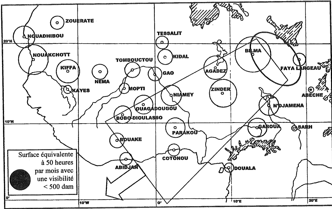
Fig.IV.51 - Fréquence annuelle des lithométéores en Afrique de l'Ouest de 1970 à 1973. Zone source décrite par BERTRAND et al. ainsi que direction des nuages (d'après BERTRAND et al. 1979, modifié).
