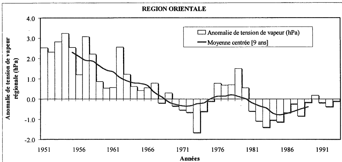
Fig.VI.9 - Evolution régionale en saison sèche (octobre à avril) de la tension de vapeur (hPa) durant la période 1951-1996. Ecarts de températures calculés par rapport à la moyenne 1961-1990 suivant l'équation III. 2. Les stations utilisées sont présentées à la figure VI. 4.
