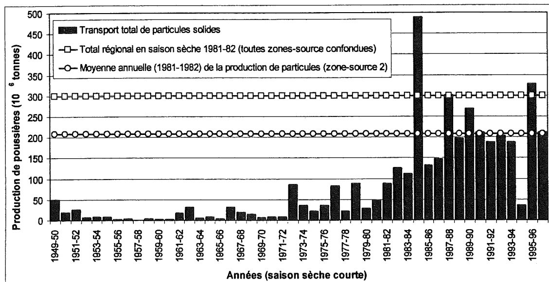
Fig.IV.72 - Transport total de particules solides ( 10^6 tonnes) de 1949 à 1996 durant la saison sèche courte (novembre à mars) à la station de Tombouctou. Comparaison est faite avec la moyenne annuelle (1981-1982) de la production de poussière de la zone source 2 ( 208 \cdot 10^6 tonnes) ainsi qu'avec le total régional (toutes zones sources confondues) estimé par D'ALMEIDA (1986) pendant la saison sèche courte 1981-82. La faible valeur observée en 1994 s'explique par le manque de données tri-horaires disponibles (1 à 2 enregistrements par jour) à cause de la rébellion touareg.
