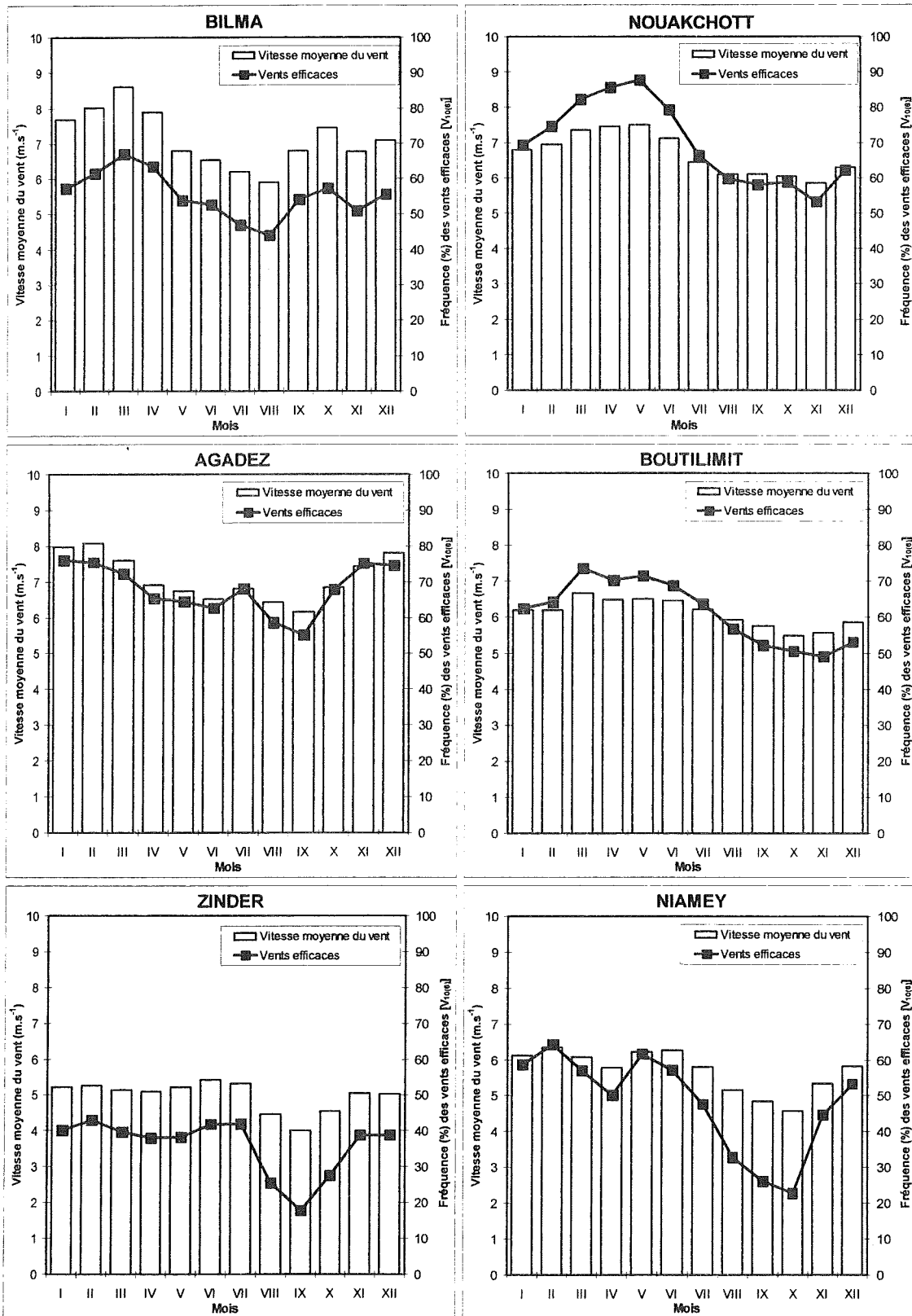
Fig.V.14 - Répartition mensuelle du vent moyen et de la fréquence des vents efficaces [V 10(6) ] observés en différentes stations (classées de la plus aride à la plus humide). Période utilisée pour les moyennes : 1951-1998, à l'exception de Nouakchott et Boutilimit (1951-1994).
