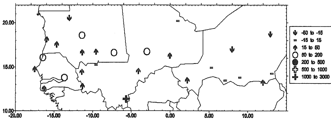
Fig.IV.41 - Evolution de la différence relative des lithométéores entre les périodes "actuelle" (1987-1997) et de sécheresse (1969-1986). La légende présente l'évolution (en %) entre ces deux périodes.
