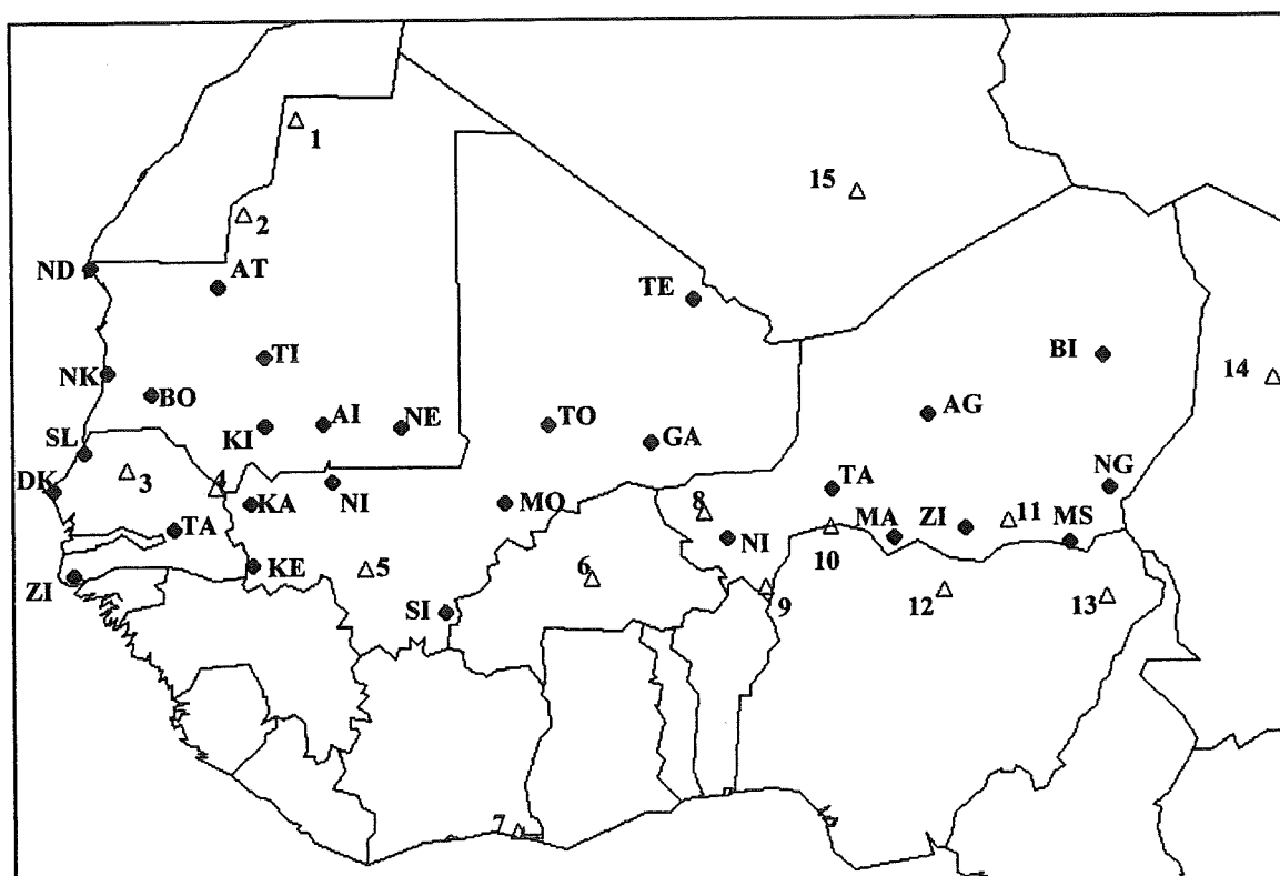
Fig.IV.33 - Répartition spatiale des stations synoptiques (●) utilisées dans cette étude pour l'analyse de l'évolution des lithométéores durant la saison sèche. Les stations numérotées (Δ) sont citées dans ce chapitre.
