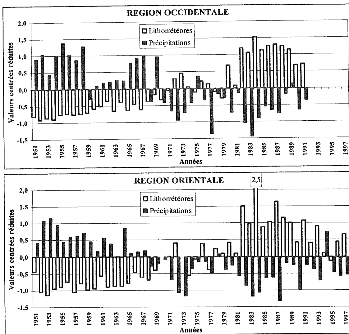
Fig.IV.59 - Evolution des précipitations et des lithométéores en saison sèche (octobre – avril) de 1951 à 1997 dans les régions occidentale et orientale de la zone d'étude. Les deux paramètres sont traduits en valeurs centrées réduites suivant la méthode de LAMB (1982).
