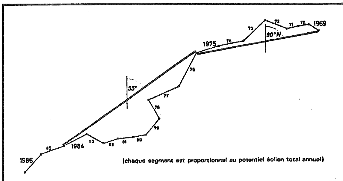
Fig.V.6 - Variations interannuelles de la résultante des vents à Tombouctou de 1969 à 1986 (COUREL & CHAMARD 1988).
