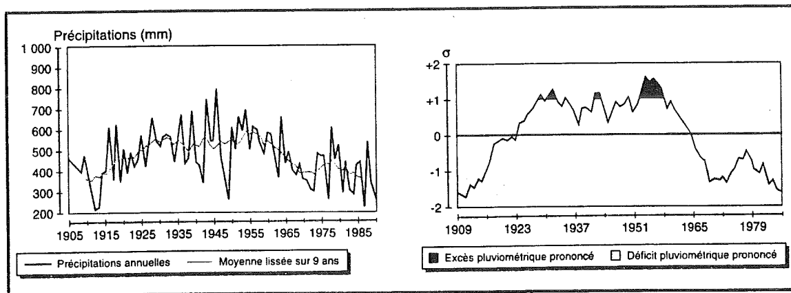
Fig.II.2 - Evolution de la pluviométrie à Zinder (Niger). A gauche, précipitations annuelles et moyenne lissée sur 9 ans de 1905 à 1990 et, à droite, courbe lissée sur 9 ans en rapport avec son écart-type (moyenne = 475 mm, écart-type = 69 mm) (OZER & ERPICUM 1995).
