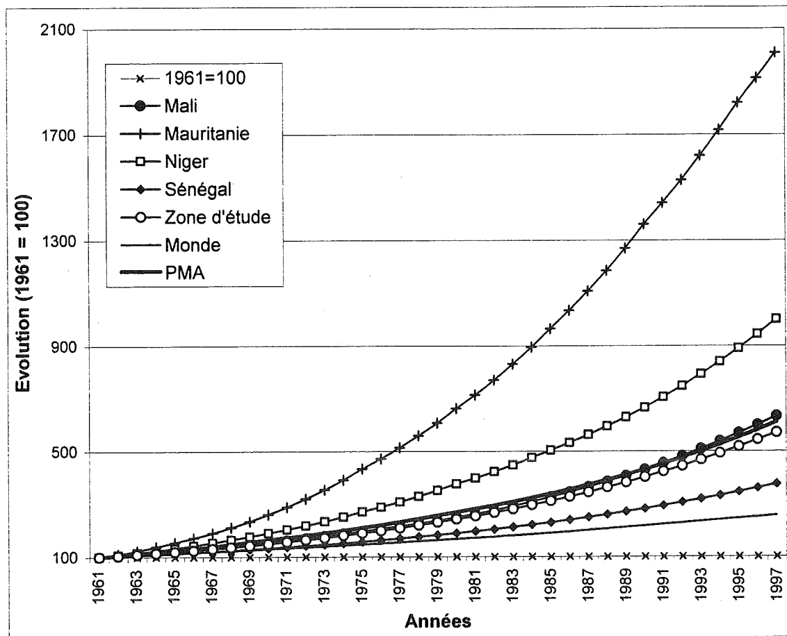
Fig.II.7. - Evolution proportionnelle de la population urbaine dans la zone d'étude de 1961 à 1997 (1961 = 100) (1961 [ 10^6 d'individus]: Niger = 0.19; Mali = 0.51; Mauritanie = 0.06; Sénégal = 1.05; PMA = 23.80; Monde = 1048.43) (d'après les données FAO, 1998).
