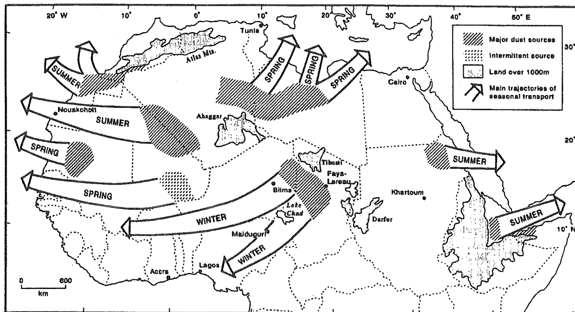
Fig.IV.1. - Principales sources de lithométéores en Afrique au nord de l'équateur et direction du transport suivant les saisons (d'après MIDDLETON 1986 in GOUDIE 1996).
