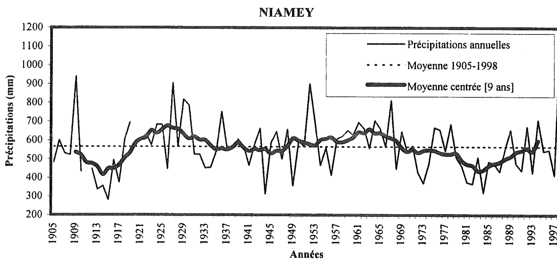
Fig.III.2 - Evolution annuelle des précipitations à Niamey de 1905 à 1998. Yearly rainfall evolution in Niamey from 1905 to 1998.
