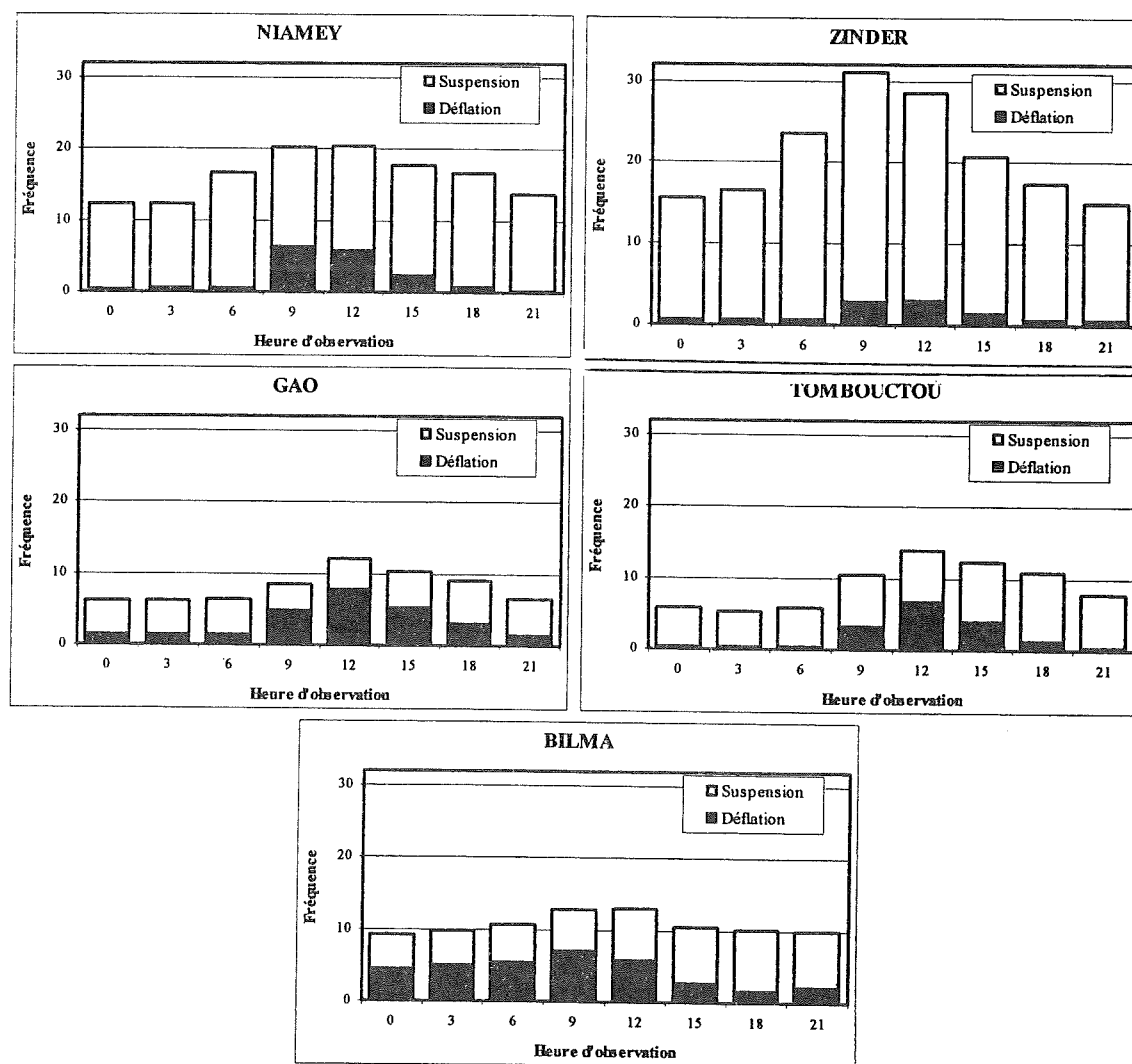
Fig.IV.21 - Fréquence moyenne (%) tri-horaire de la visibilité réduite par les lithométéores à moins de 500 dam durant la saison sèche (novembre à mars). Les données utilisées pour ces calculs couvrent la période 1947-1997.
