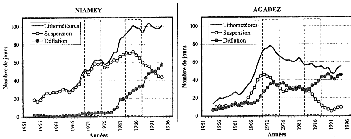
Fig.IV.50 - Evolution (moyenne centrée sur 7 ans) des lithométéores, suspension et déflation aux stations d'Agadez et Niamey de 1951 à 1997. Les cases indiquent les deux périodes analysées par N'TCHAYI et al. (1994, 1997)
