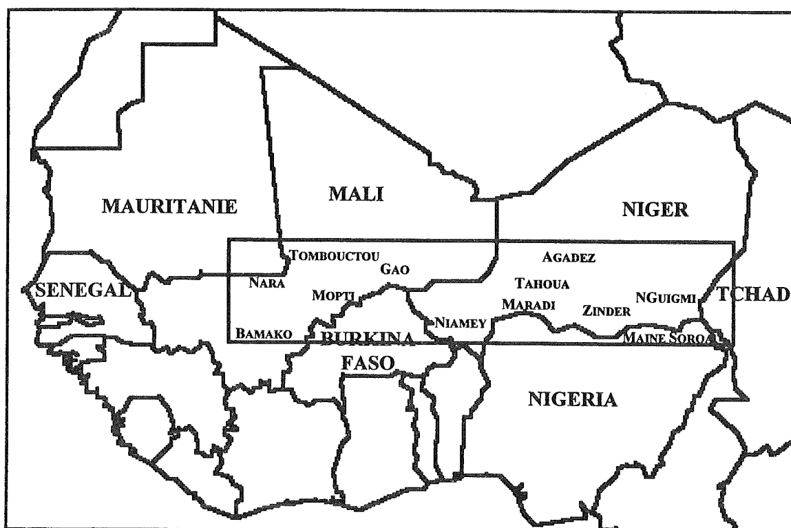
Fig.IV.28 - Localisation de la zone présentée ci-après à la figure IV. 29 (fenêtre 8°00W,17°00N – 15°00E,12°30N)
