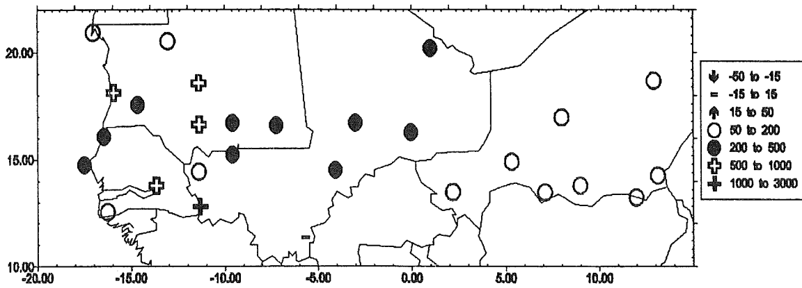
Fig.IV.40 - Evolution de la différence relative des lithométéores entre les périodes de sécheresse (1969-1986) et "humide" (1951-1968). La légende présente l'évolution (en %) entre ces deux périodes.
