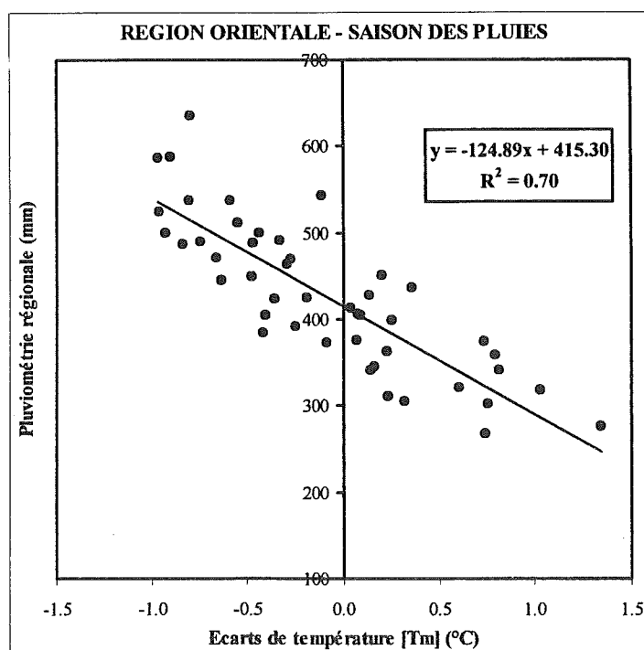
Fig. VI.7 - Relation entre la pluviométrie régionale (mm) et les écarts de température moyenne (°C). Relation between regional rainfall (mm) and mean temperature (°C).
