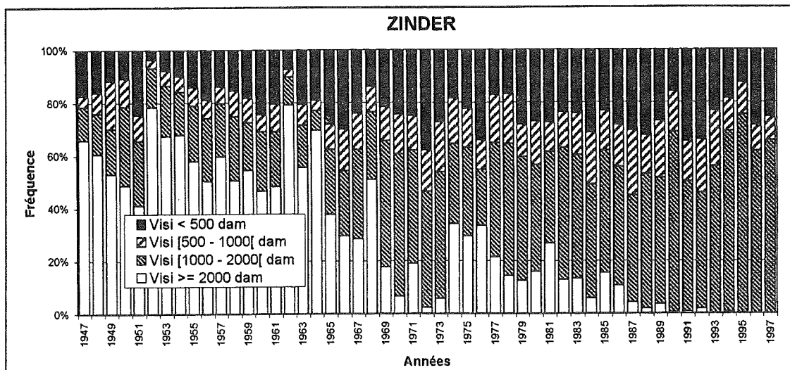
Fig.IV.20 - Répartition des visibilités à la station synoptique de Zinder durant la saison sèche (novembre à mars) de 1947 à 1997. Les données tri-horaires sont utilisées pour le calcul de la fréquence.
