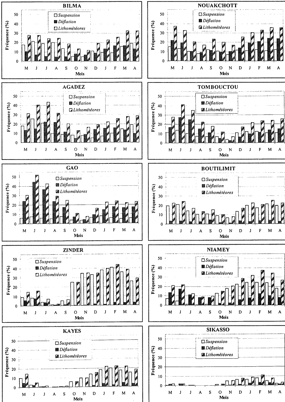
Fig.IV.27 - Répartition mensuelle (de mai à avril) des lithométéores (suspension, déflation et total) observés en différentes zones caractéristiques de la région d'étude (classées du plus aride au plus humide) Période utilisée pour les moyennes: 1951-1997, à l'exception de Nouakchott et Boutilimit (1951-1994).
