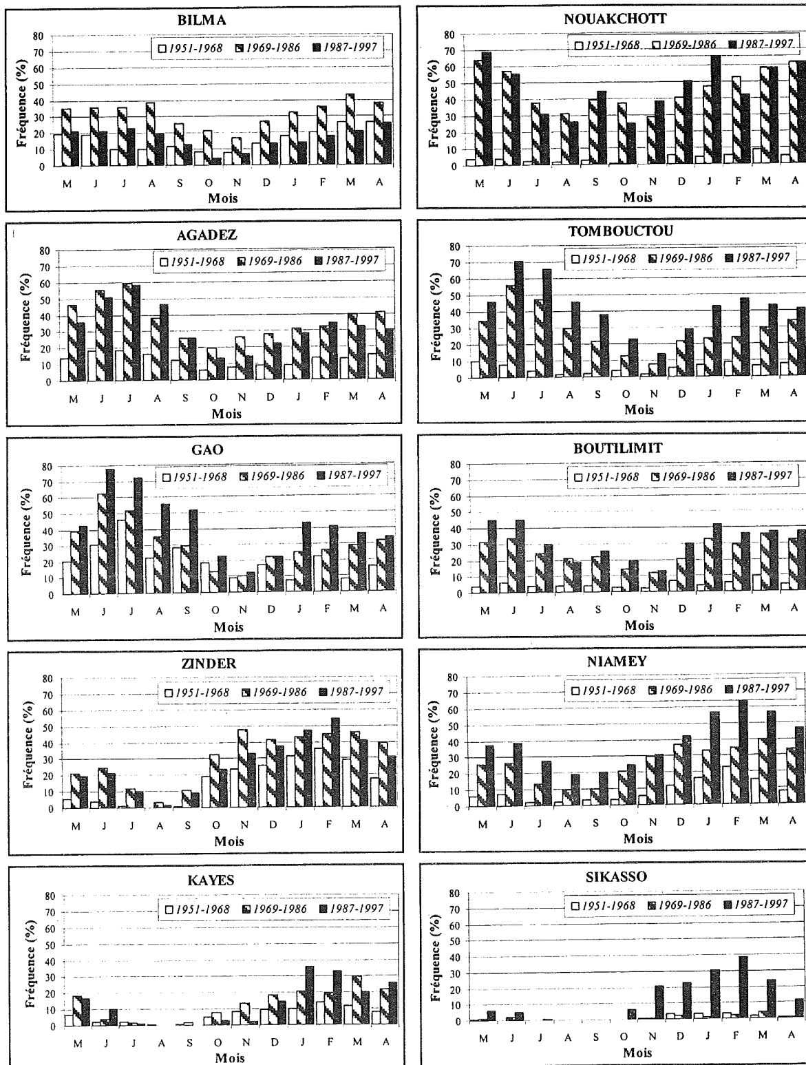
Fig.IV.30 - Répartition mensuelle (de mai à avril) des lithométéores observés en différentes stations synoptiques de la région d'étude (classées du plus aride au plus humide) pour les périodes "humide", (1951-1968), de sécheresse (1969-1986) et "actuelle" (1987-1997).
