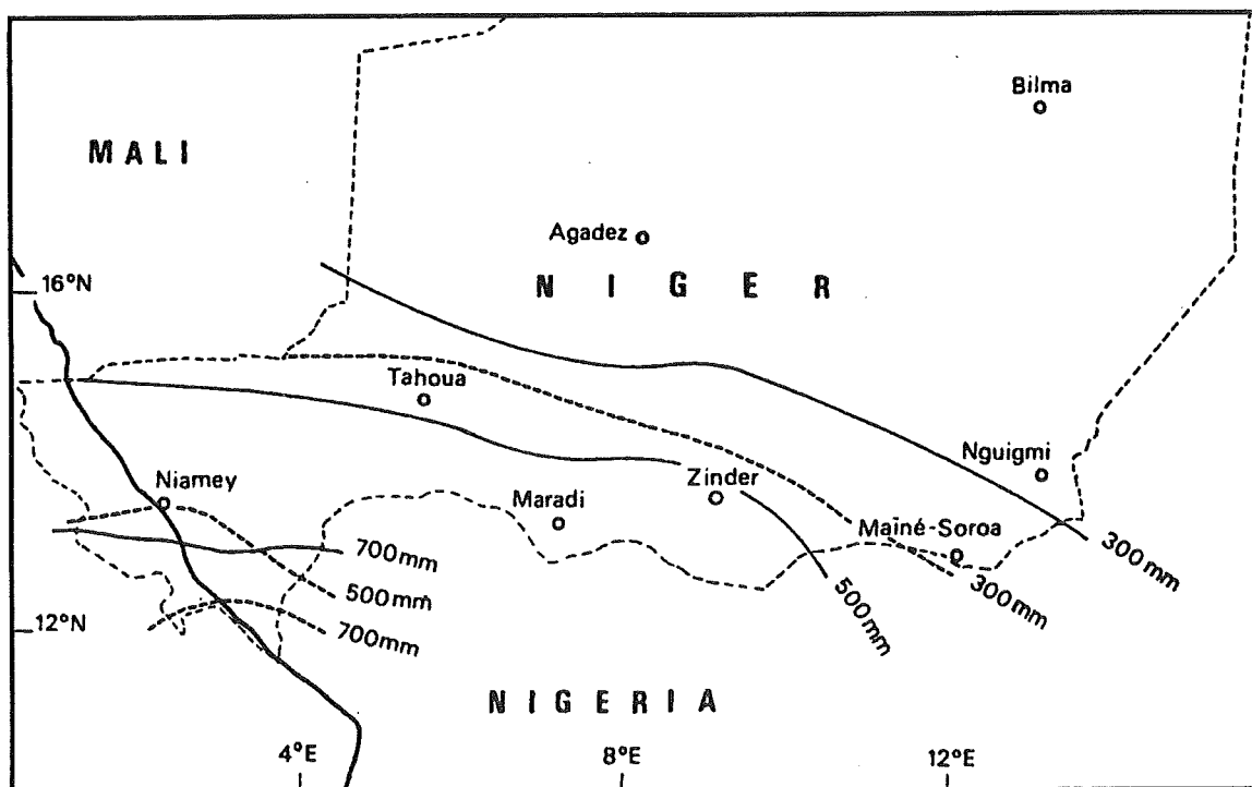
Fig.IV.15 - Carte de localisation des stations synoptiques utilisées par OZER (1998) pour l'étude de l'évolution de la fréquence des lithométéores au Niger. Les isohyètes sont établis pour la période "humide" de 1951 à 1967 (—) et pour la période de sécheresse de 1968 à 1987 (---).
