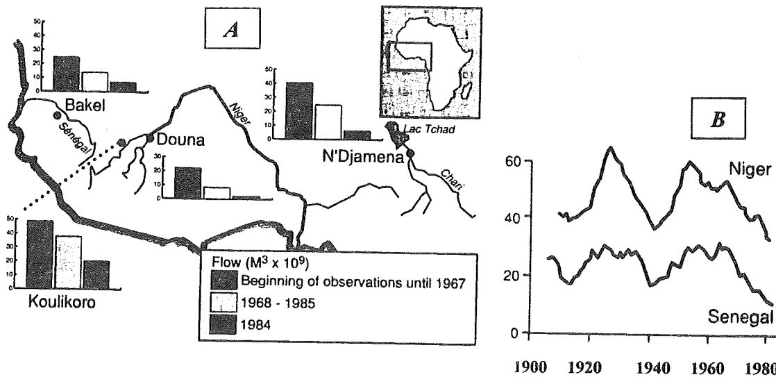
Fig.II.3 - Variations récentes du débit ( 10^9 \text{ m}^3 \text{ an}^{-1} ) de certains cours d'eau importants au Sahel (A) et moyenne lissée sur 7 ans du débit des fleuves Niger et Sénégal (B). (d'après WALLING, 1996).
