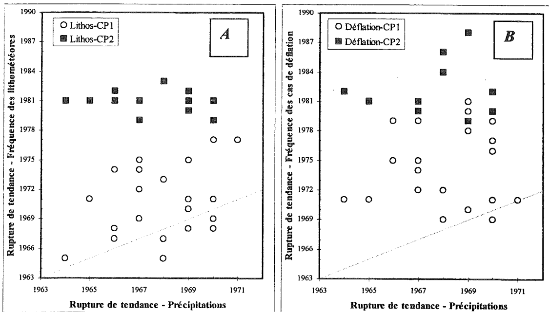
Fig.IV.54 - Relation entre les années des points de rupture de tendance calculés par le test de PETTITT (1979) pour les séries pluviométriques et [A] la fréquence de lithométéores et [B] la fréquence des cas de déflation. CP1: premier point de rupture, CP2: deuxième point de rupture.
