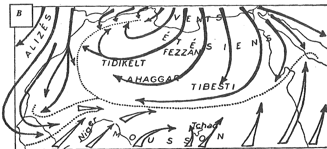
Figure.V.1. - Direction des vents prédominants sur l'Afrique de l'Ouest en janvier [A] et en juillet [B] (d'après DUBIEF 1952).
