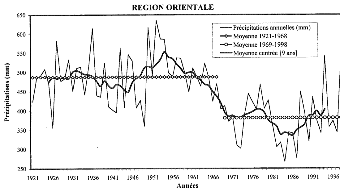
Fig.III.6 - Précipitations régionales annuelles et moyenne des sous-séries pluviométriques avant et après le point de rupture de 1968.
