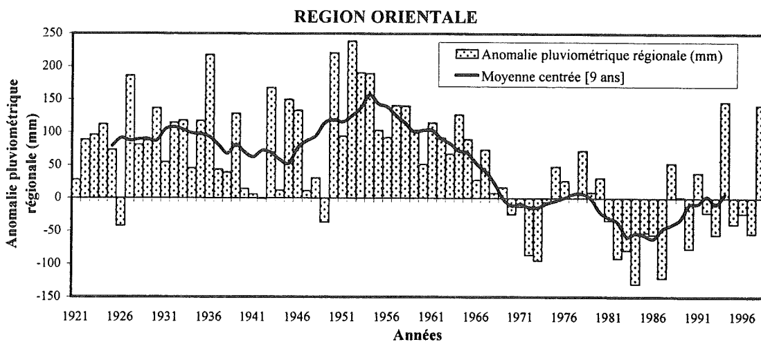
Fig.III.5 - Evolution de l'anomalie pluviométrique régionale (Mali et Niger) exprimée en mm, par rapport à la moyenne de la période 1961-1990 (397 mm), de 1921 à 1998 dérivée de l'Eq.III.2 (JONES & HULME 1996).
