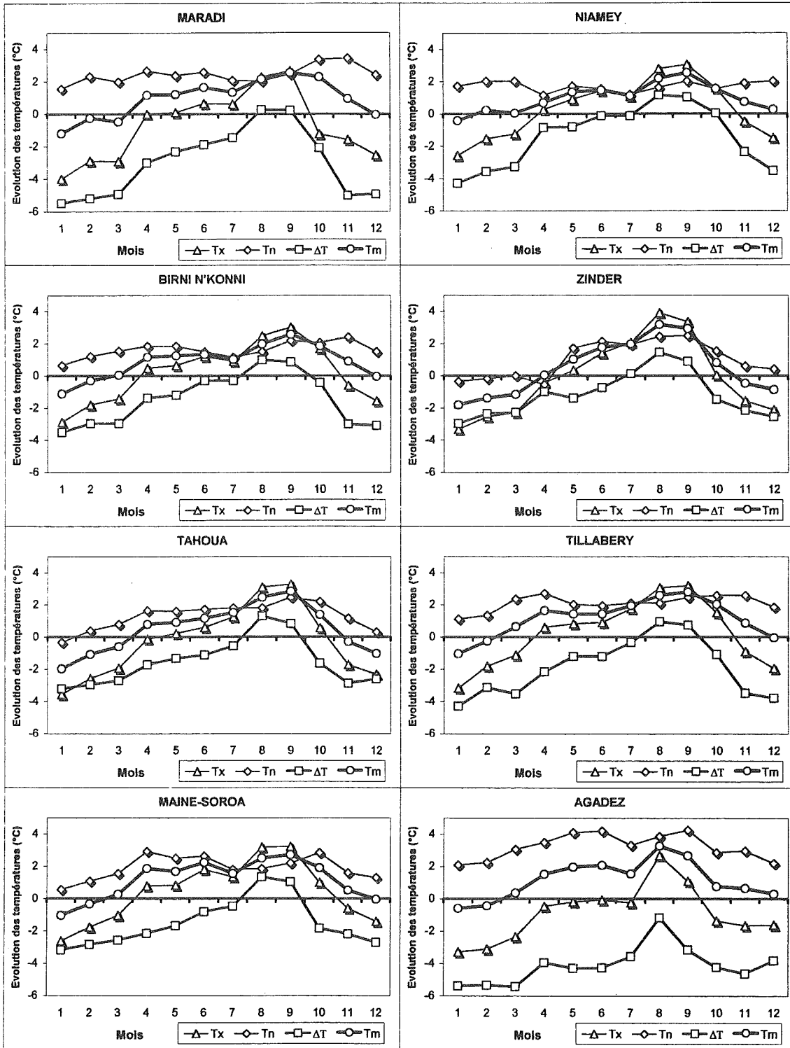
Fig.VI.3 - Tendances des températures maximales (Tx), minimales (Tn), moyennes (Tm) et des amplitudes thermiques diurnes ( \Delta T ) moyennes mensuelles calculées sur la période 1951-1993 en huit stations nigériennes.
