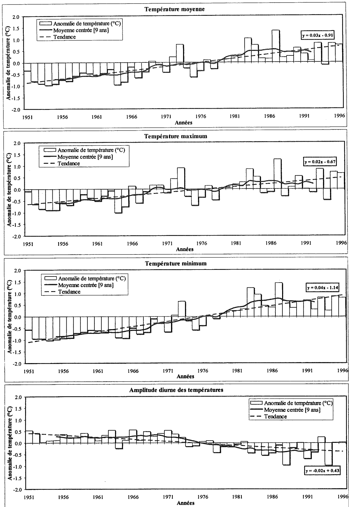
Fig.VI.6 - Evolution régionale en saison des pluies (mai à septembre) des températures moyennes, maximales, minimales et des amplitudes thermiques diurnes moyennes durant la période 1951-1996. Ecarts de températures calculés par rapport à la moyenne 1961-1990 suivant l'équation III. 2.
