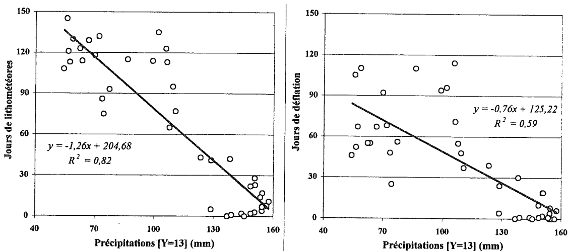
Fig.IV.56 - Relation maximum entre la fréquence [A] des lithométéores et [B] des cas de déflation avec la pluviométrie moyenne des années (Y=13) précédentes à Nouakchott.
