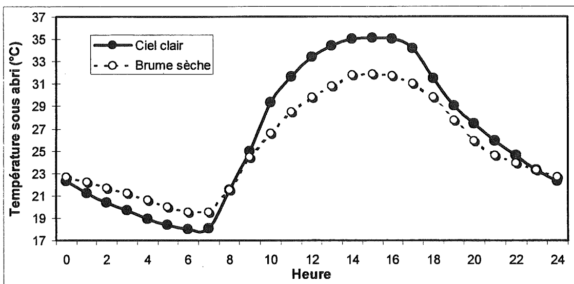
Fig. VI.10 - Températures horaires moyennes mesurées sous abri à Niamey en situation de ciel clair ( VV > 1500 dam) et en situation de brume sèche ( VV < 500 dam) (d'après MODI 1983).
