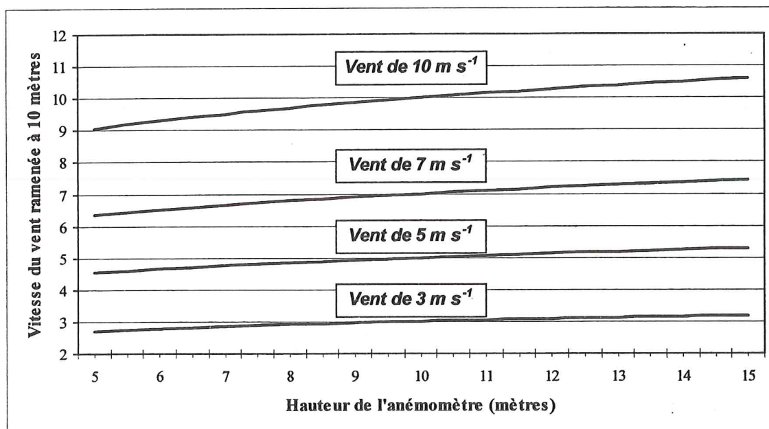
Fig.V.4 - Fluctuation, obtenue à partir de l'application de la formule [Eq. 1], de la vitesse d'un vent de 3, 5, 7 et 10 \text{ m s}^{-1} mesurée à dix mètres au dessus du sol en fonction de la hauteur de l'anémomètre.
