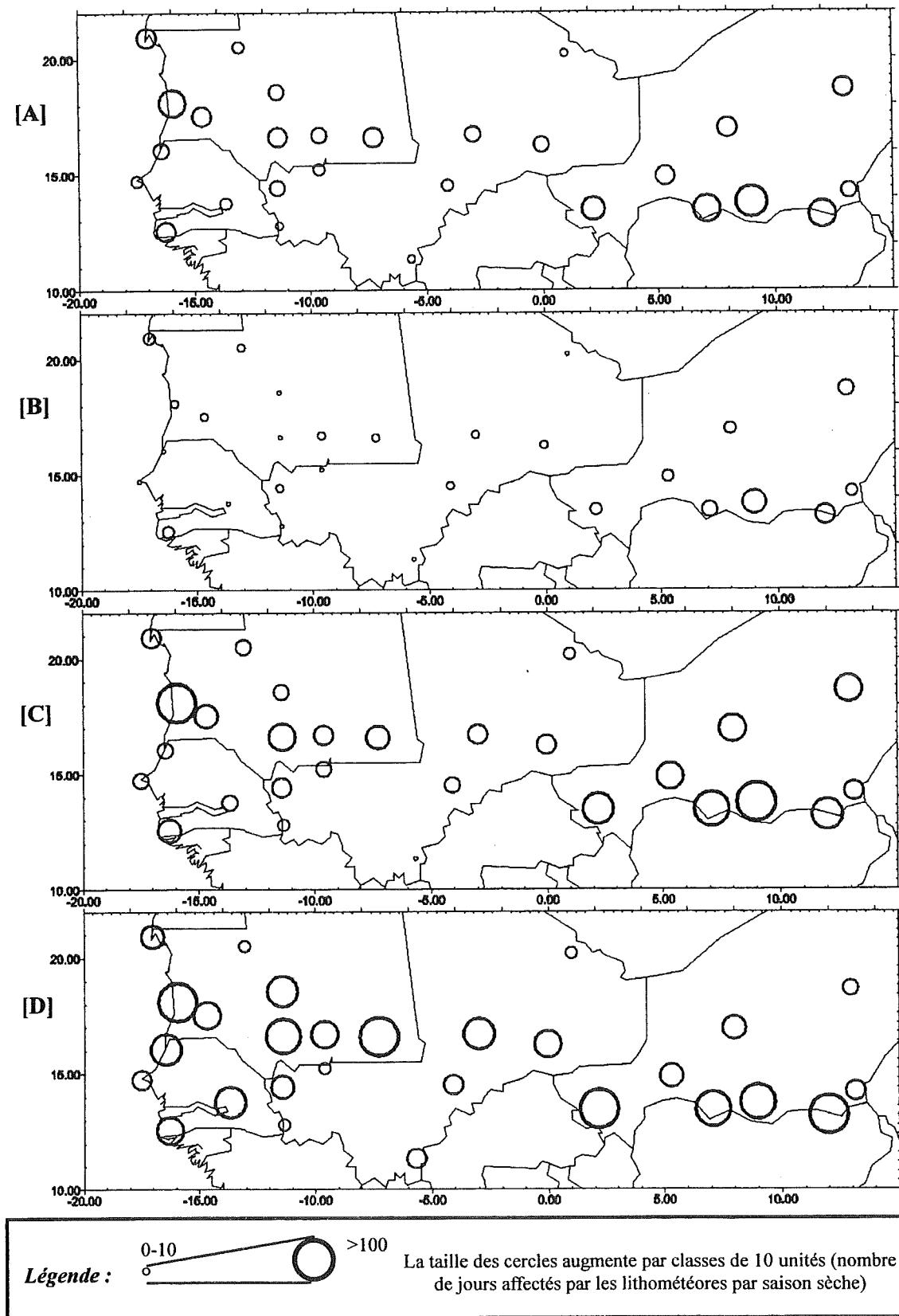
Fig.IV.39 - Répartition des lithométéores durant [A] la période 1947-1997, et pour les périodes [B] "humide" (1951-1968), [C] de sécheresse (1969-1986) et [D] "actuelle" (1987-1997).
