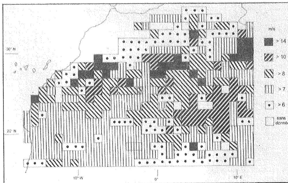
Fig.V.8 - Vitesse minimum du vent efficace définie par degré carré à dix mètres au dessus du sol. (d'après MARTICORENA et al. 1997).
