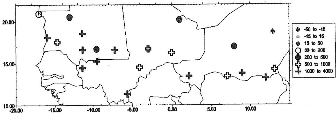
Fig.IV.49 - Evolution de l'occurrence des cas de déflation entre les périodes "actuelle" (1987-1997) et "humide" (1951-1968). La légende présente l'évolution (en %) entre ces deux périodes. Evolution of the deflation frequency between the "present" (1987-1997) and the "humid" (1951-1968) periods. The legend shows the evolution (%) between these two periods.
