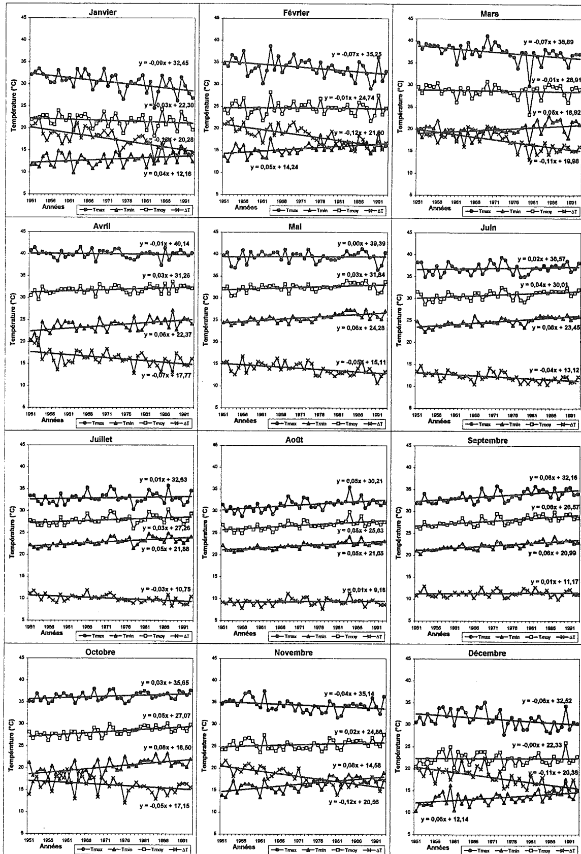
Fig.VI.2 - Evolution mensuelle des températures maximales (Tx), minimales (Tn), moyennes (Tm) et de l'amplitude thermique diurne (ΔT) à la station de Maradi durant la période 1951-1993.
