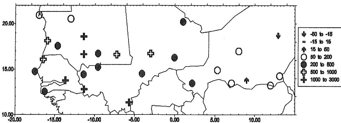
Fig.IV.42 - Evolution de la différence relative des météores entre les périodes "actuelle" (1987-1997) et "humide" (1951-1968). La légende présente l'évolution (en %) entre ces deux périodes.
