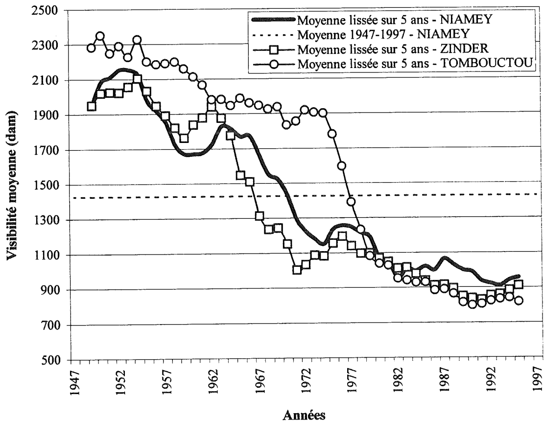
Fig.IV.18 - Visibilité moyenne (saison sèche - novembre à mars) observée aux stations synoptiques de Niamey, Zinder et Tombouctou de 1947 à 1997. Données tri-horaires.
