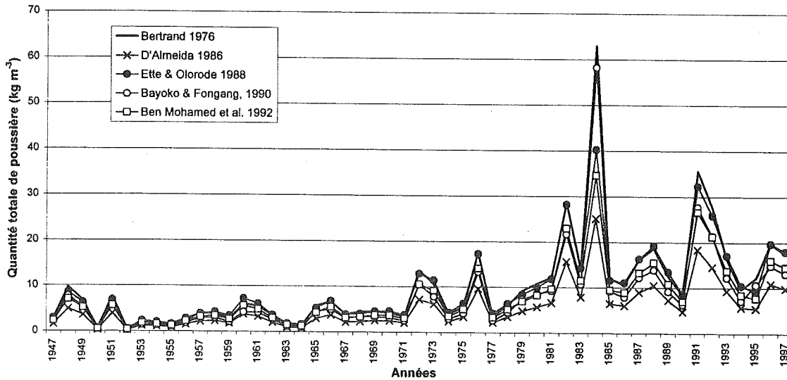
Fig.IV.67 - Cf. Fig. IV.65 uniquement pour les visibilitées tri-horaires inférieures à 500 dam. Moyenne 1947-1997: BERTRAND (1976): 10.1; D'ALMEIDA (1986): 5.4; ETTE et OLORODE (1988): 9.6; BAYOKO et FONGANG (1990): 7.9; BEN MOHAMED et al. (1992): 7.8.
