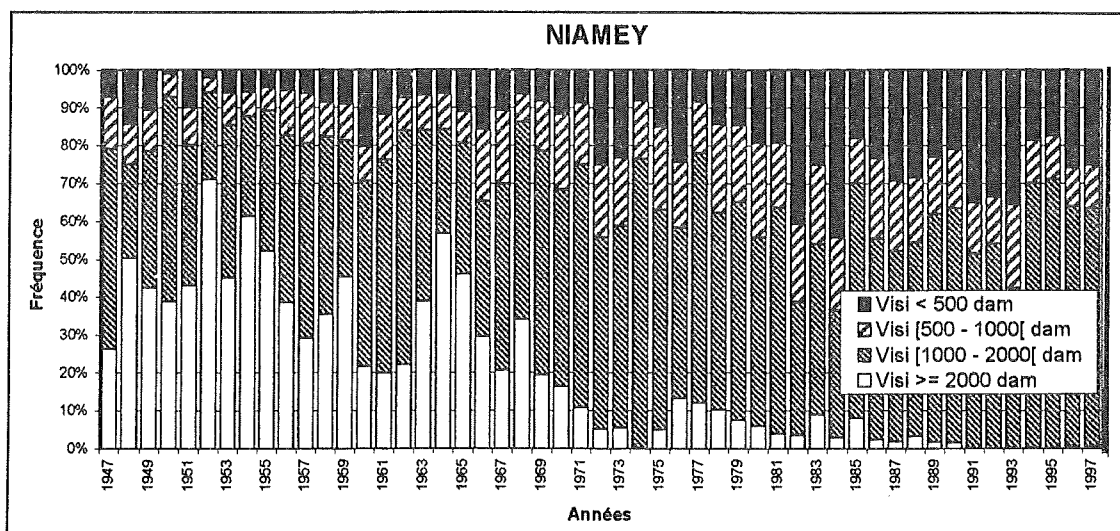
Fig.IV.19 - Répartition des visibilités à la station synoptique de Niamey durant la saison sèche (novembre à mars) de 1947 à 1997. Les données tri-horaires sont utilisées pour le calcul de la fréquence (1208 cas par saison sèche).
