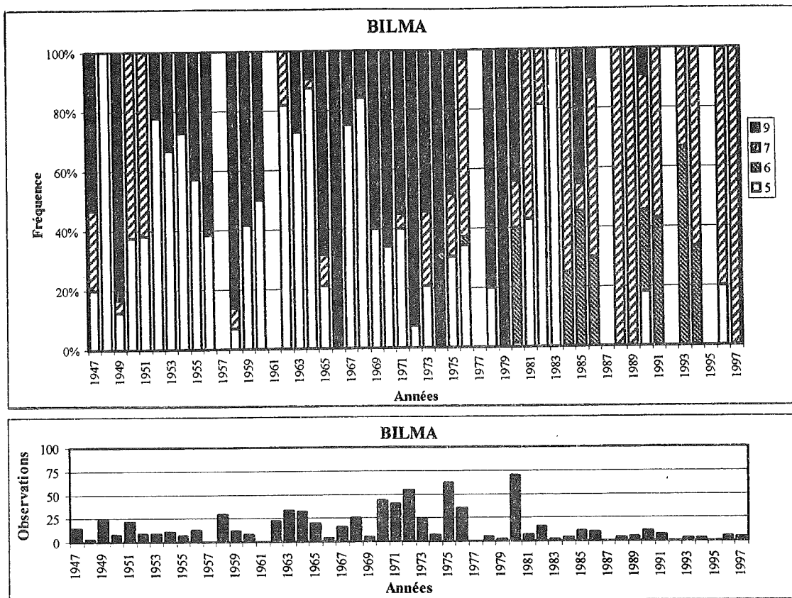
Fig.IV.9 - Répartition des types de lithométéores réduisant la visibilité à moins de 100 dam, observés aux stations synoptiques de Niamey, Zinder, Gao, Tombouctou et Bilma durant la saison sèche (novembre à mars) de 1947 à 1997. Légende: (5) brume sèche; (6) brume de poussière; (7) chasse-sable; (9) tempête de sable. (5) et (6) correspondent au transport simple (suspension) de particules solides, et (7) et (9) à la déflation. Les colonnes blanches indiquent l'absence de lithométéores réduisant la visibilité à moins de 100 dam. A la suite de ces représentations, les bâtonnets montrent le nombre d'observations (tri-horaires) prises en compte pour le calcul de la fréquence.
