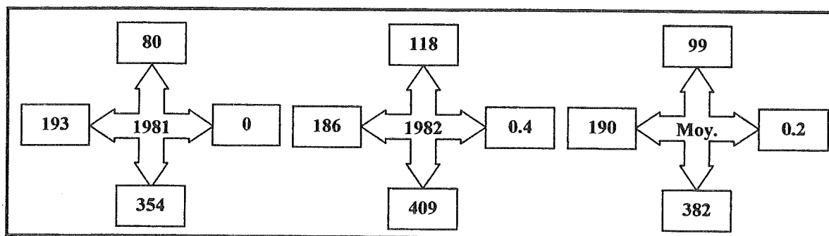
Fig.IV.69 - Production de poussières estimée en millions de tonnes (total des quatre zones sources) suivant les directions en 1981, 1982 et en moyenne d'après D'ALMEIDA (1986).
