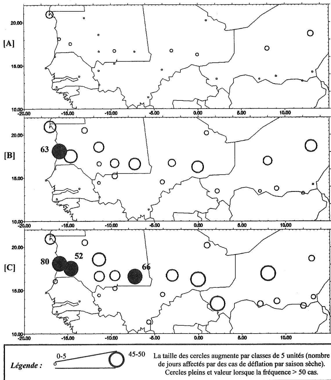
Fig.IV.46 - Répartition des cas de déflation durant les périodes [A] "humide" (1951-1968), [B] de sécheresse (1969-1986) et "actuelle" (1987-1997).
