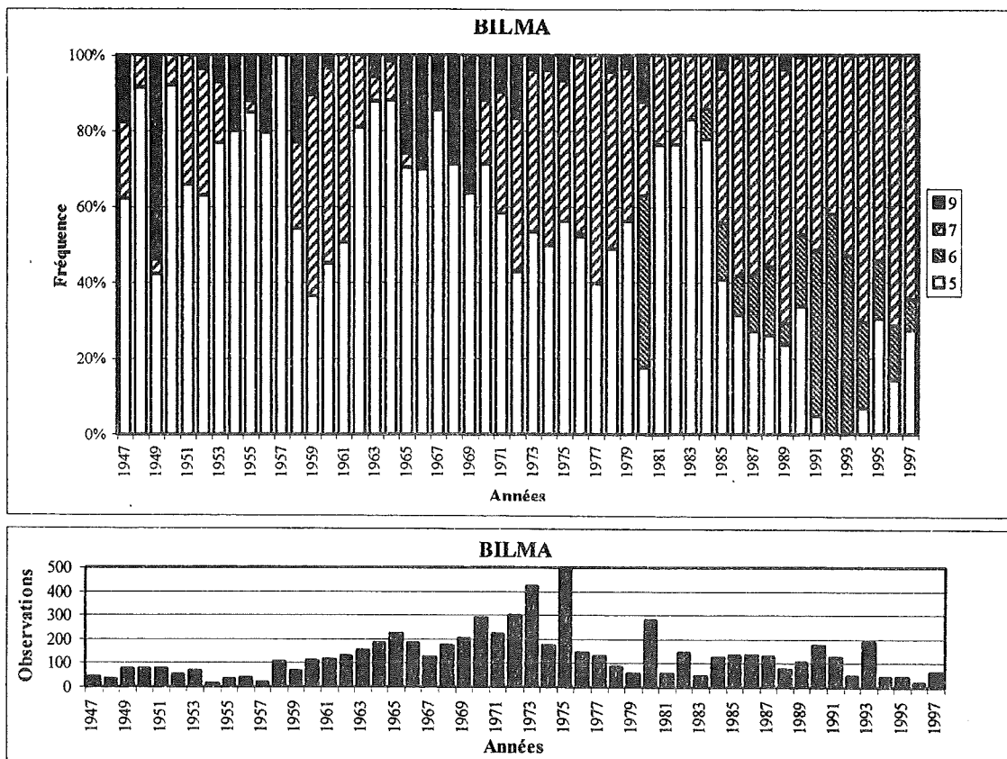
Fig.IV.10 - Répartition des types de lithométéores réduisant la visibilité à moins de 500 dam, observés aux stations synoptiques de Niamey, Zinder, Gao, Tombouctou et Bilma durant la saison sèche (novembre à mars) de 1947 à 1997. Légende: (5) brume sèche; (6) brume de poussière; (7) chasse-sable; (9) tempête de sable. (5) et (6) correspondent au transport simple (suspension) de particules solides, et (7) et (9) à la déflation. Les colonnes blanches indiquent l'absence de lithométéores réduisant la visibilité à moins de 100 dam. A la suite de ces représentations, les bâtonnets montrent le nombre d'observations (tri-horaires) prises en compte pour le calcul de la fréquence.
