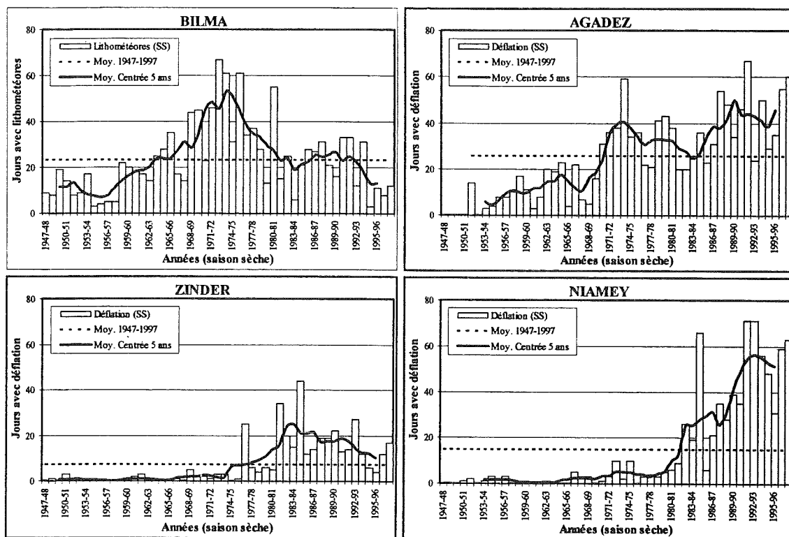
Fig.IV.43 - Evolution des cas de déflation en saison sèche (octobre - avril) au Niger de 1947-48 à 1997-98. La courbe moyenne (pointillés) détermine la période utilisée pour chaque station.
