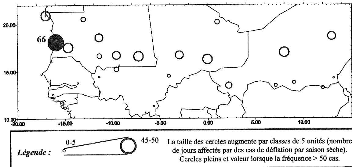
Fig.IV.45 - Répartition des cas de déflation durant la période 1947-1997.
