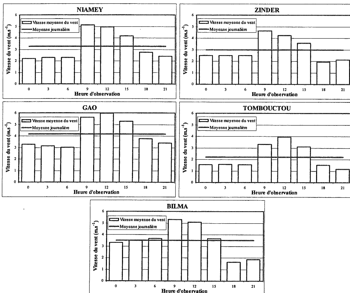
Fig.V.10 - Vitesse moyenne tri-horaire du vent durant la saison sèche (novembre à mars). Les données utilisées pour ces calculs couvrent la période 1947-1997, sauf pour Bilma (1954-1997), Gao (1950-1996) et Tombouctou (1949-1996).
