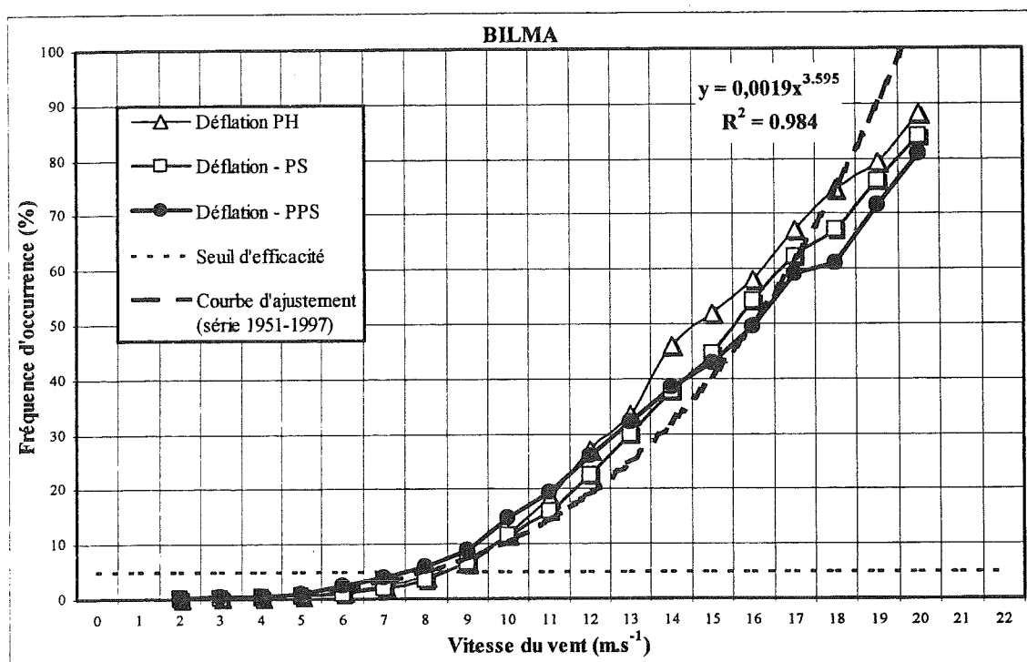
Fig.V.26 - Evolution de la fréquence d'observation des jours avec déflation en fonction de la vitesse du vent (m s -1 ). Comparaison entre les périodes "humide" (PH: 1951-1968), de sécheresse (PS: 1969-1986) et "actuelle" (PPS : 1987-1997). La courbe d'ajustement est appliquée à toutes les données (1951-1997).
