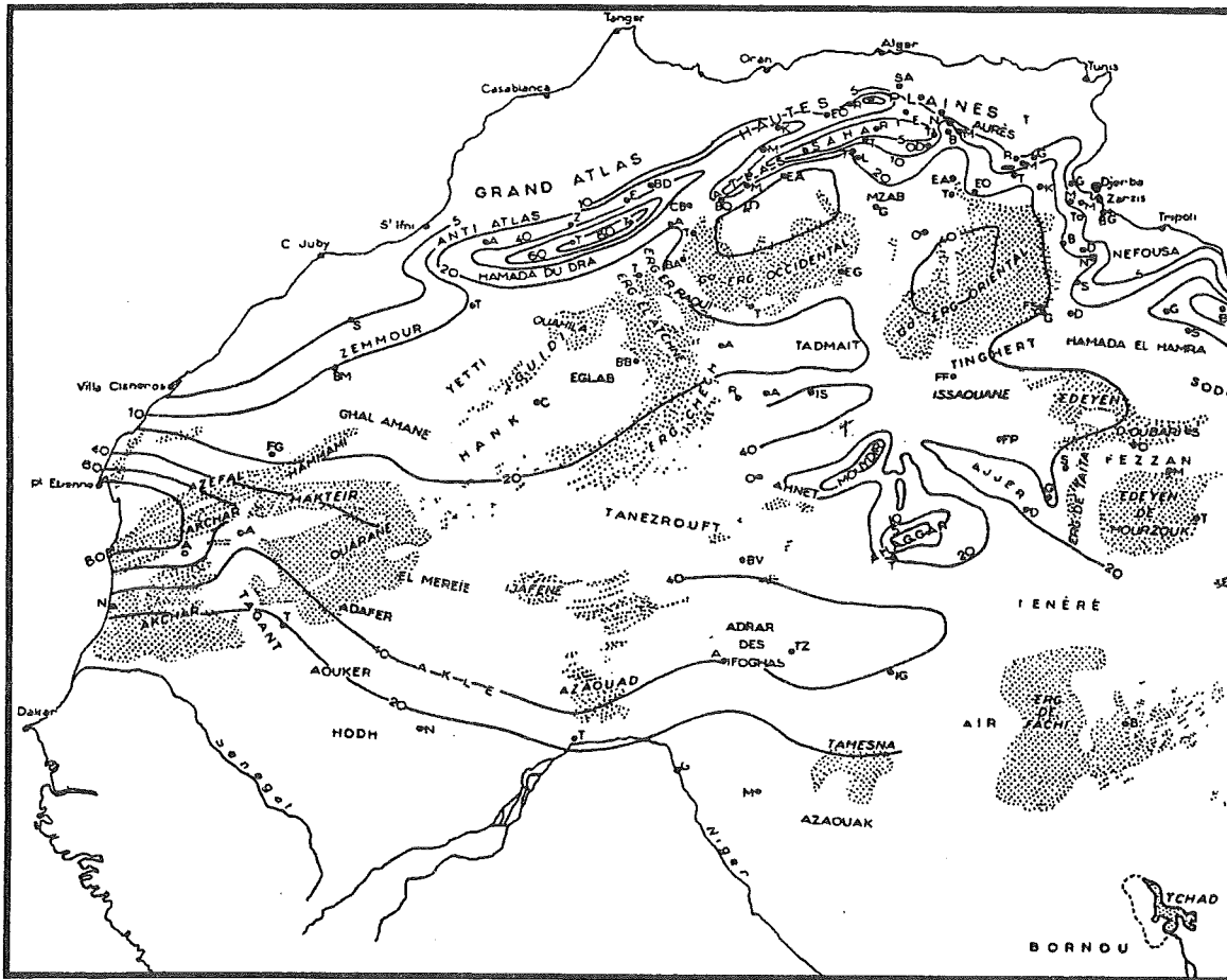
Fig.IV.12. - Répartition géographique des lithométéores (vents de sable) dans le Sahara et ses bordures de 1925 à 1950 (d'après DUBIEFF 1952).
