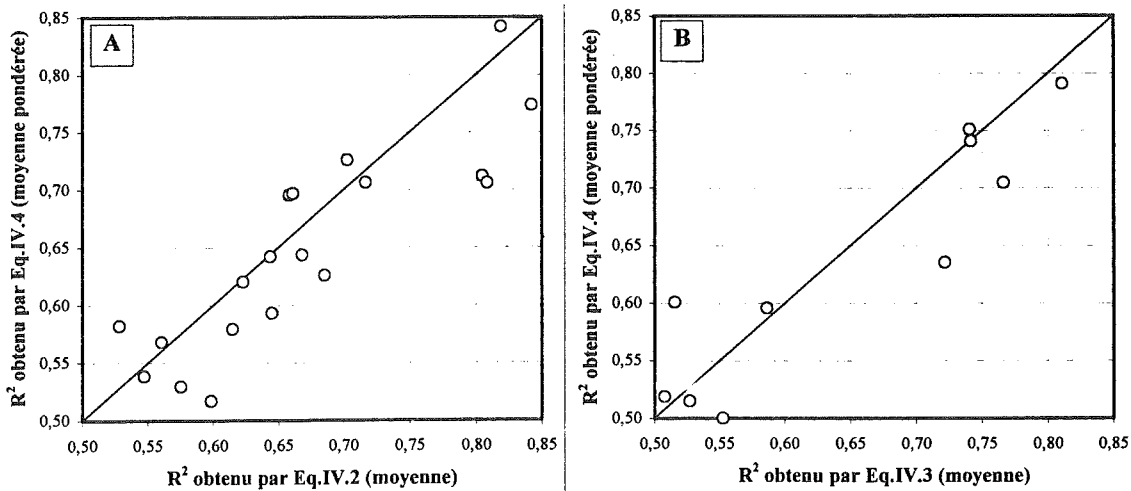
Fig.IV.57 - Relation entre les coefficients de détermination maximum dérivés des équations IV. 2, IV. 3 et IV. 4 liant la pluviométrie moyenne et la pluviométrie moyenne pondérée à [A] la fréquence des lithométéores et [B] la fréquence des cas de déflation.
