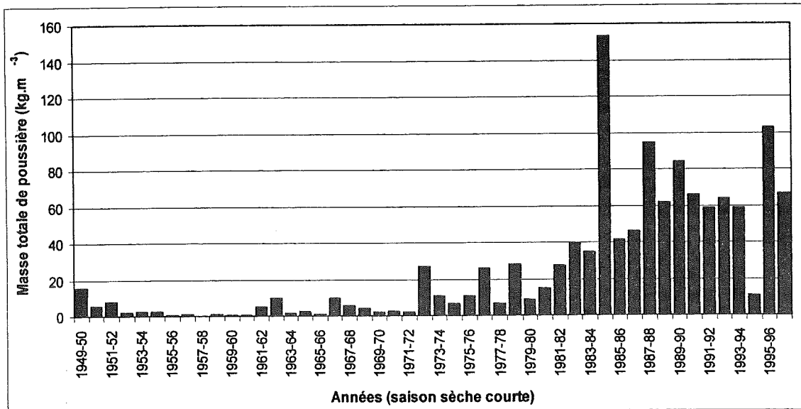
Fig.IV.71 - Transport total de particules solides ( \text{kg.m}^{-3} ) obtenu pour une surface verticale de 1 \text{ m}^2 à une hauteur de dix mètres au-dessus du sol, de 1949 à 1996 durant la saison sèche courte (novembre à mars) à la station de Tombouctou.
