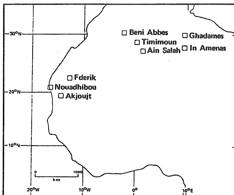
Fig.V.5 - Carte de localisation des stations météorologiques utilisées par HELGREN et PROSPERO (1987). Location of the stations used by HELGREN and PROSPERO (1987).
