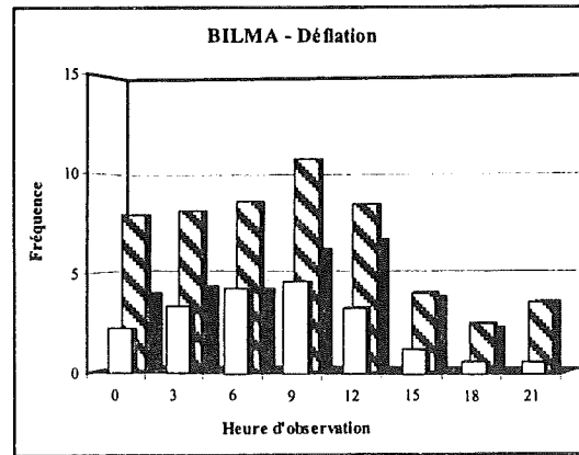
Fig.IV.26 - Fréquence moyenne (%) tri-horaire de la visibilité réduite par les poussières en suspension et les cas de déflation durant la saison sèche (novembre à mars) à la station de Bilma. Comparaison entre les périodes "humide" (1951-1968, blanc), de sécheresse (1969-1986, hachuré), et "actuelle" (1987-1997, noir).
