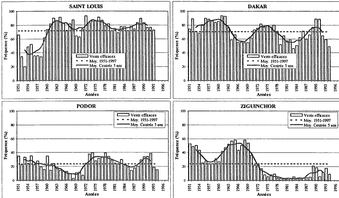
Fig.V.16 - Evolution annuelle de la fréquence des vents efficaces [V_{10(6)}] au Sénégal de 1951 à 1994.
