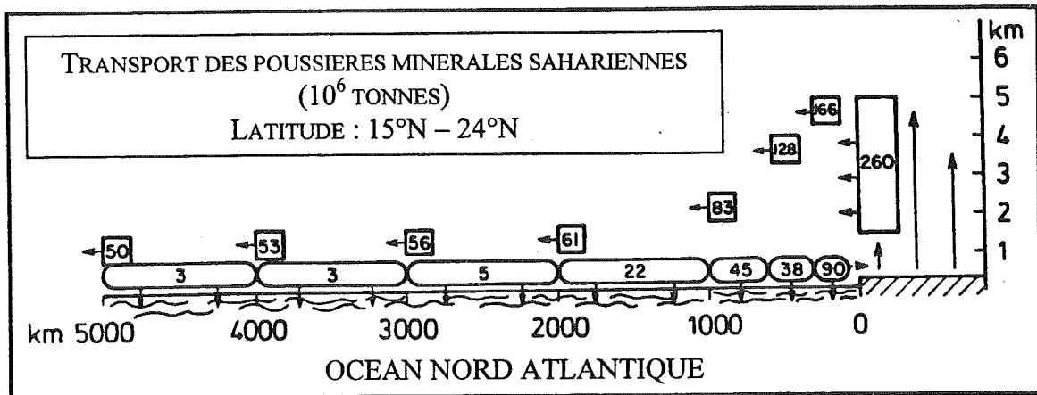
Fig.IV.3. - Budget annuel de poussières transportées depuis les côtes de l'Afrique de l'Ouest (0 km) vers les Barbades (4500 km) (d'après SCHUTZ et al. 1981).
