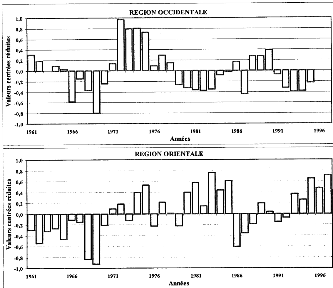
Fig.V.19 - Evolution de la fréquence des jours enregistrant des vents efficaces [ V_{10(6)} ] de 1961 à 1997 dans les régions occidentale et orientale de la zone d'étude. Le paramètre est traduit en valeurs centrées réduites suivant la méthode de LAMB (1982).
