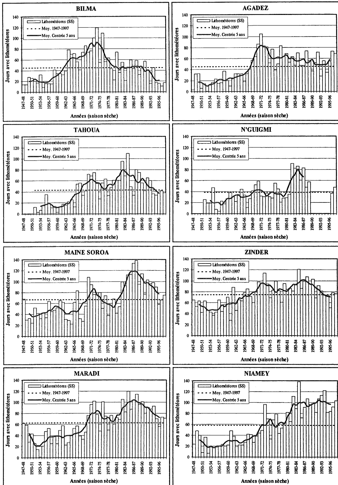
Fig.IV.34 - Evolution du nombre de jours affectés par les lithométéores en saison sèche (octobre – avril) au Niger de 1947-48 à 1997-98. La moyenne détermine la période utilisée pour chaque station.
