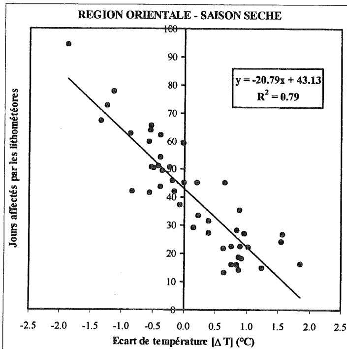
Fig.VI.12 - Relation entre la fréquence régionale des lithométéores et les écarts de l'amplitude thermique diurne (°C) régionale.
