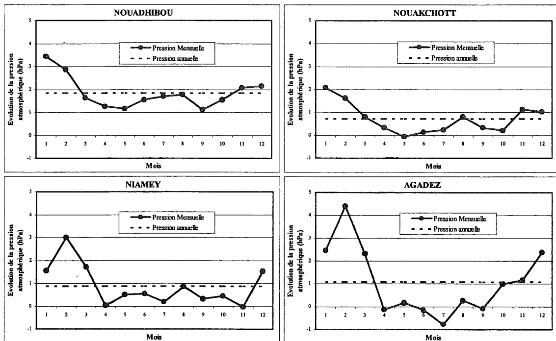
Fig.V.21 - Répartition mensuelle de l'évolution de la pression atmosphérique (hPa) en Mauritanie (Nouadhibou et Nouakchott: 1961-1994) et au Niger (Niamey et Agadez: 1968-1997).
