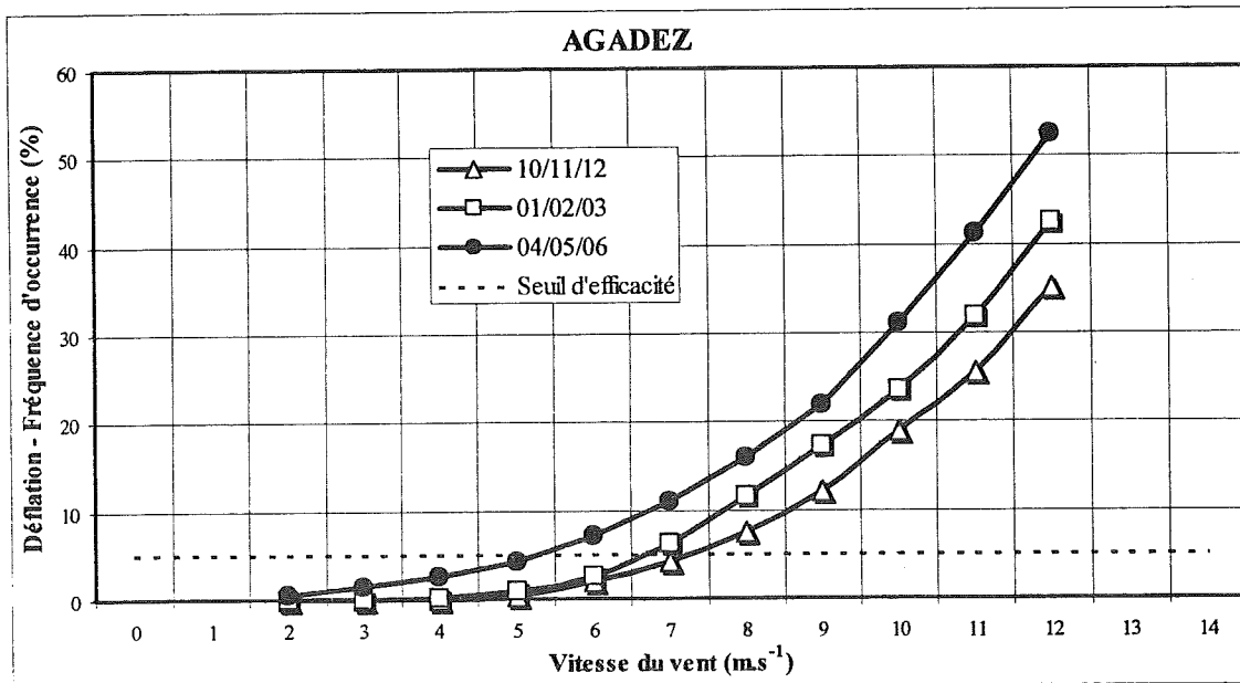
Fig.V.28 - Evolution de la fréquence d'observation des jours avec déflation en fonction de la vitesse du vent ( m s^{-1} ) à la station de Agadez de 1951 à 1997. Comparaison entre trois périodes de la saison sèche du Sahel septentrional (octobre-décembre, janvier-mars et avril-juin).
