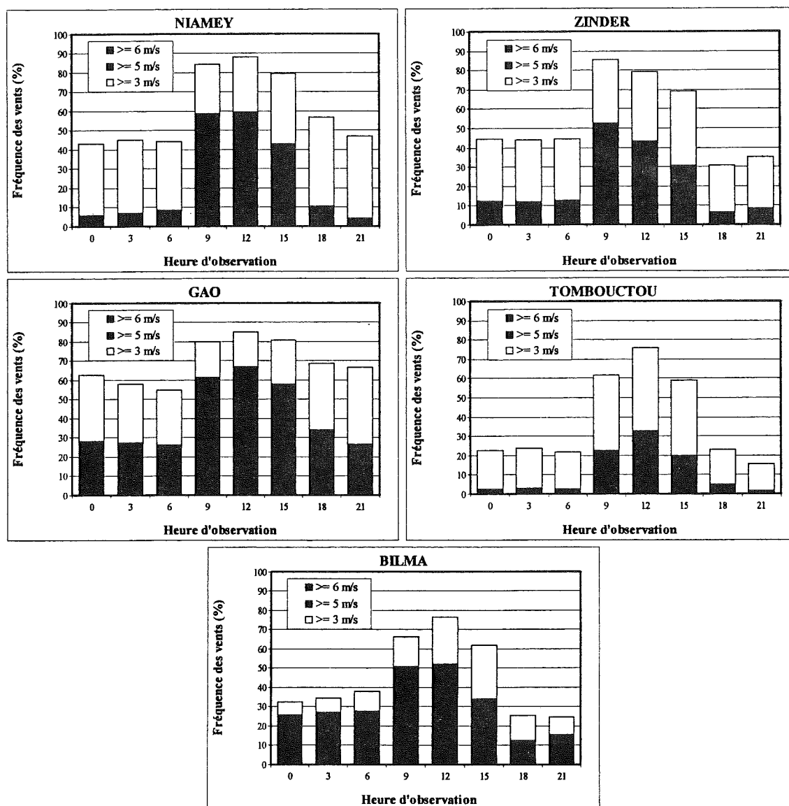
Fig.V.12 - Fréquence moyenne (%) tri-horaire des vents efficaces ( V_{10(3)} , V_{10(5)} et V_{10(6)} ) durant la saison sèche (novembre à mars). Les données utilisées pour ces calculs couvrent la période 1947-1997 sauf Bilma (1954-1997), Gao (1950-1996) et Tombouctou (1949-1996).
