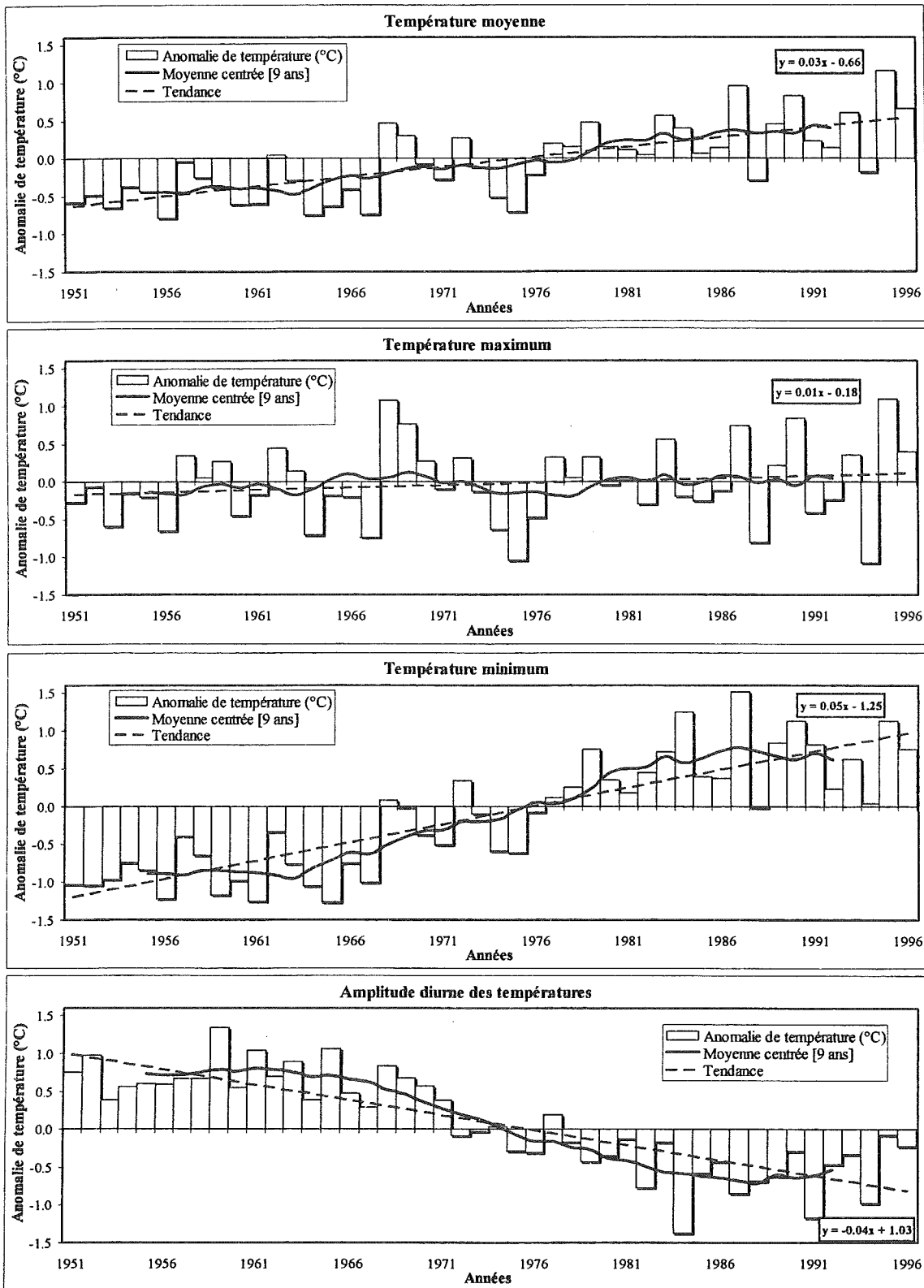
Fig.VI.5 - Evolution régionale des températures moyennes, maximales, minimales et des amplitudes thermiques diurnes moyennes annuelles durant la période 1951-1996. Les écarts de températures sont calculés par rapport à la moyenne 1961-1990 suivant l'équation III. 2.
