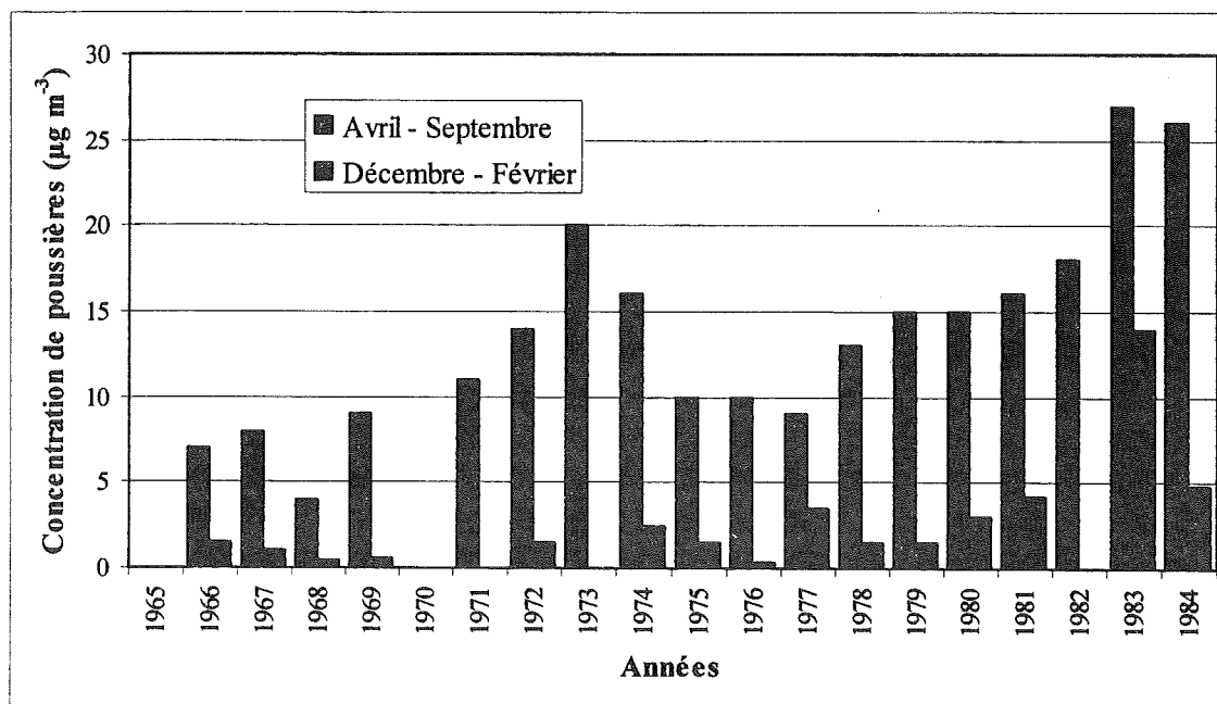
Fig.IV.4 - Concentration moyenne de poussières sahariennes en Barbade pour les mois d'avril à septembre et pour les mois de décembre à février (d'après PROSPERO & NEES 1986).
