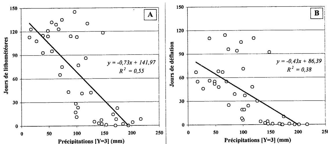
Fig.IV.55 - Relation entre la fréquence [A] des lithomètres et [B] des cas de déflation avec la pluviométrie moyenne des trois années précédentes à Nouakchott.
