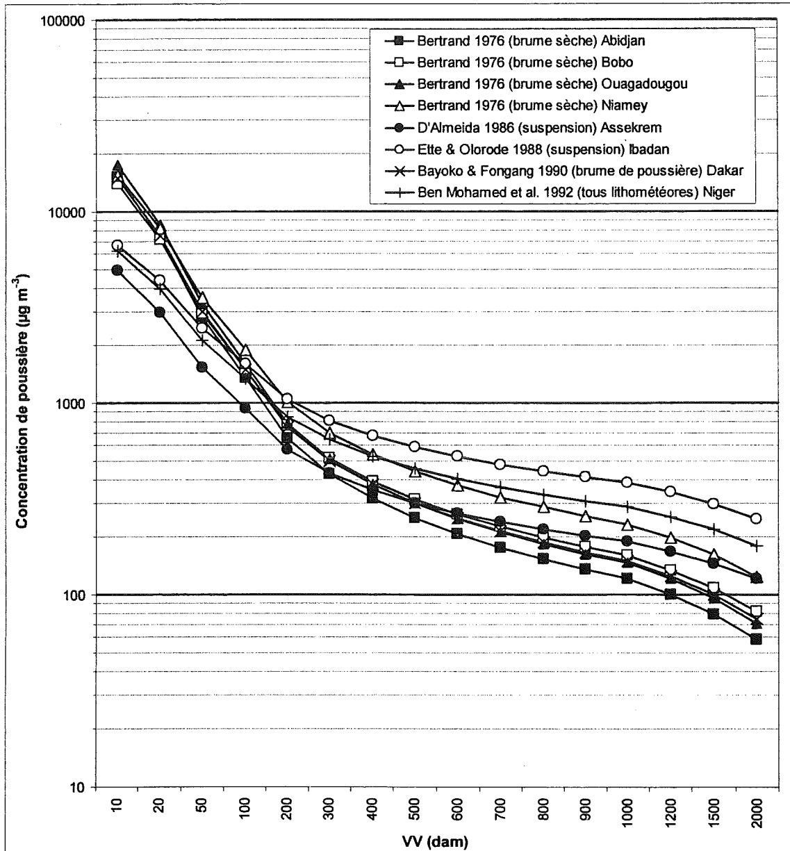
Fig.IV.64 - Relation entre visibilité et concentration en particules solides en suspension dans l'atmosphère suivant divers auteurs.
