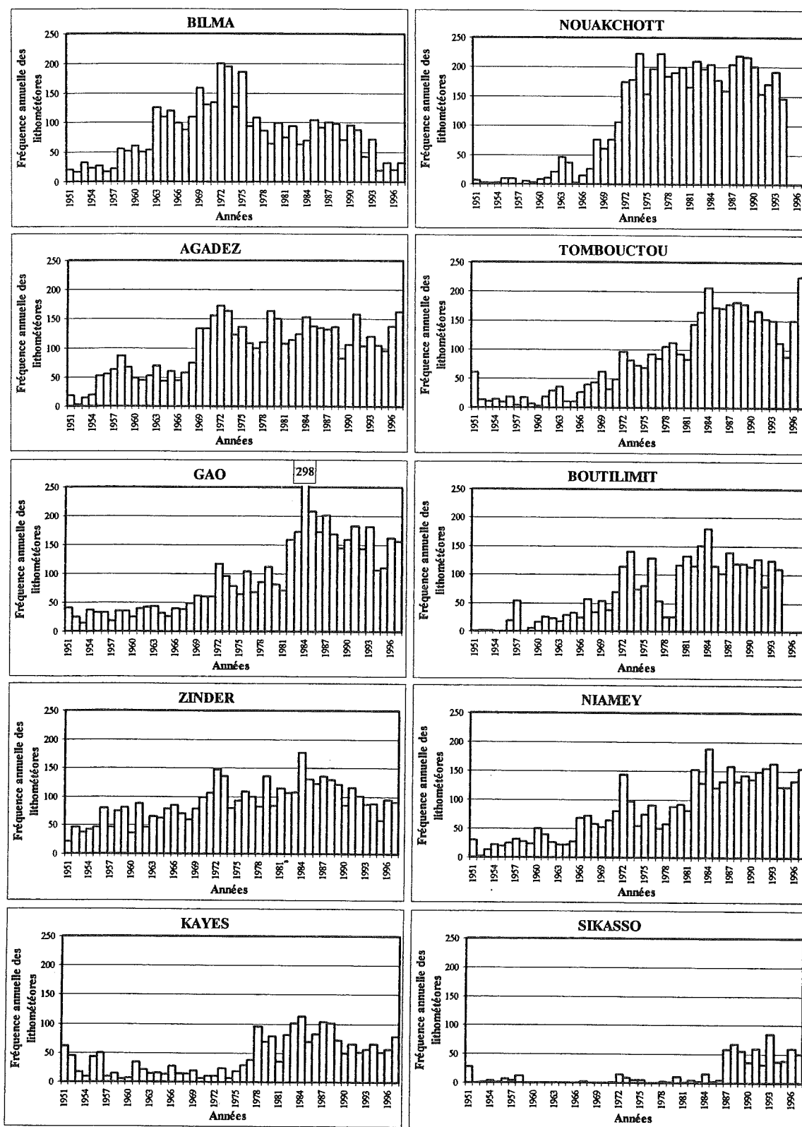
Fig.IV.32 - Evolution annuelle (mai à avril) du nombre de jours avec lithométéores observées en différentes stations caractéristiques de la région d'étude (classées du plus aride au plus humide) de 1951 à 1997 (sauf pour les stations de Nouakchott à Boutlimit: 1951-1994)
