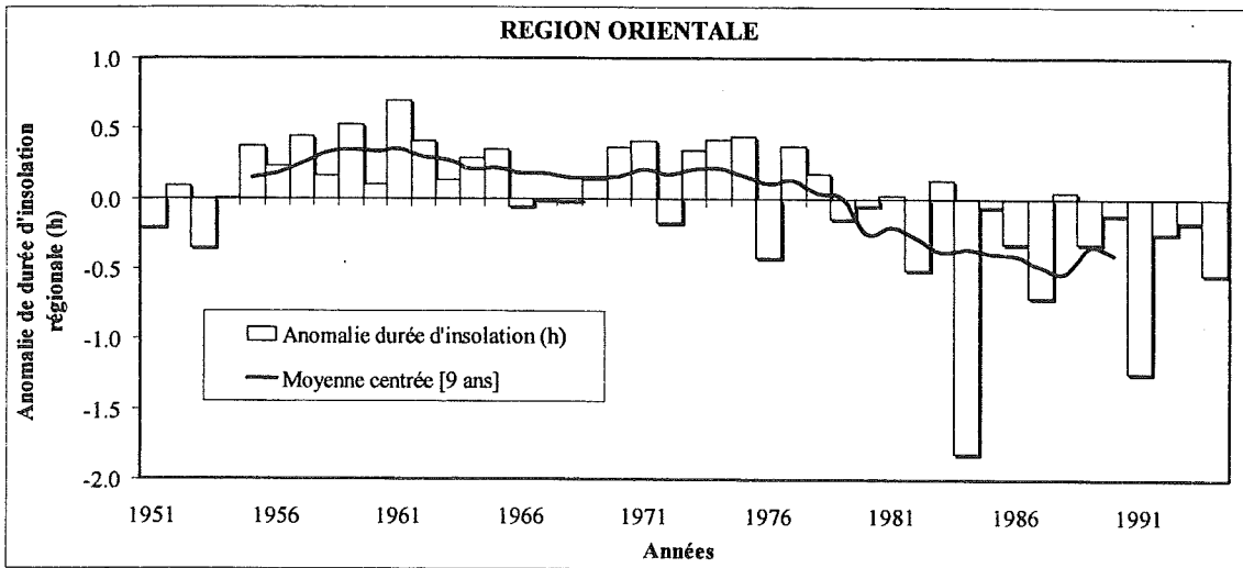
Fig.VI.11 - Evolution régionale en saison sèche (octobre à avril) de la durée d'insolation (heures) durant la période 1951-1994. Les écarts de durée d'insolation sont calculés par rapport à la moyenne 1961-1990 (9 heures) suivant l'équation III. 2. Les stations utilisées sont présentées à la figure VI. 4.
