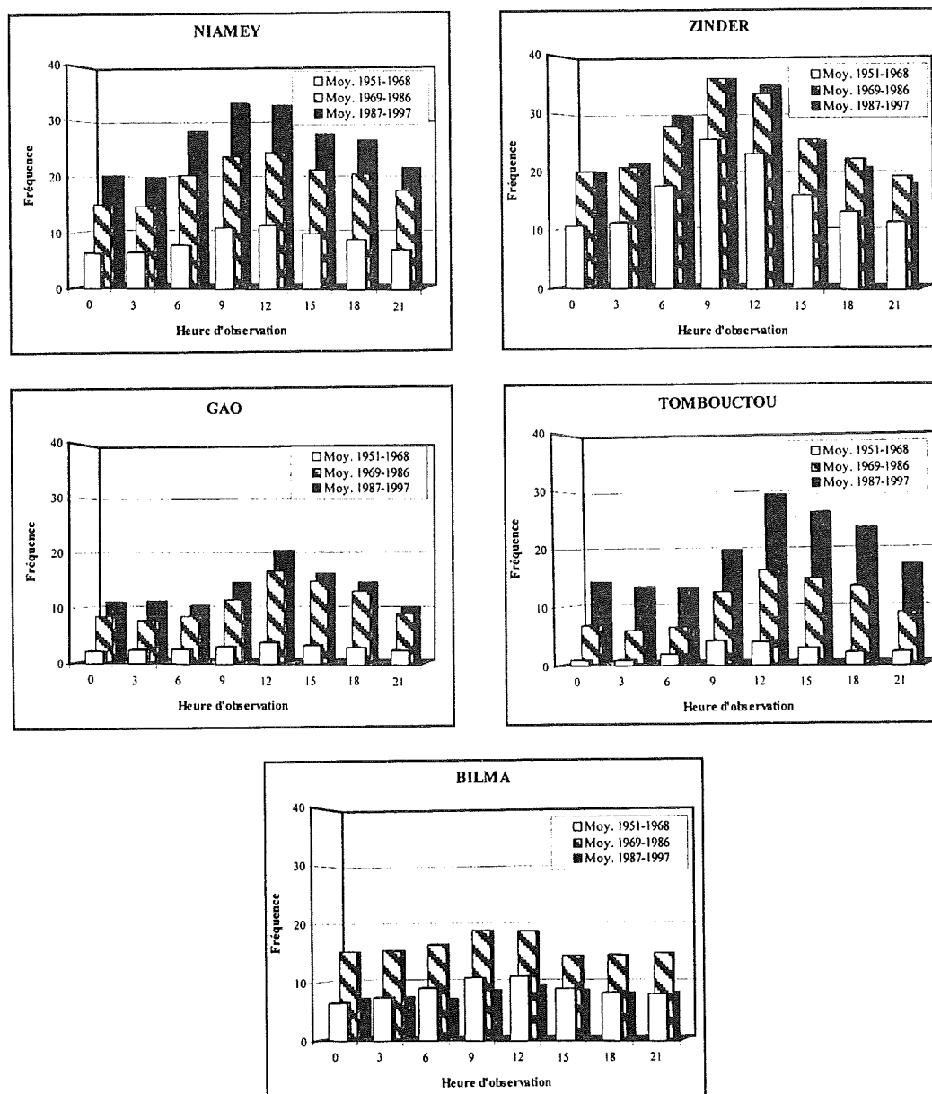
Fig.IV.22 - Fréquence moyenne (%) tri-horaire de la visibilité réduite par les lithométéores à moins de 500 dam durant la saison sèche (novembre à mars). Comparaison entre les périodes "humides" (1951-1968) de sécheresse (1969-1986) et "actuelle" (1987-1997).
