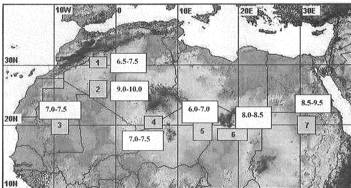
Fig.V.9 - Estimation de la vitesse minimum du vent efficace à dix mètres au dessus du sol ( m s^{-1} ) pour sept zones test dont l'extension spatiale est présentée sur fond gris (d'après CHOMETTE et al. 1999).
