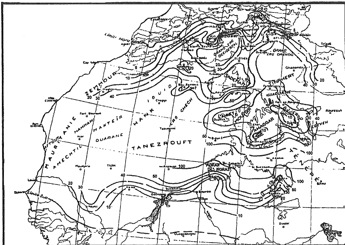
Fig.IV.11. - Répartition géographique des lithométéores (vents de sable) dans le Sahara et ses bordures de 1925 à 1939 (d'après DUBIEFF 1943). 1
