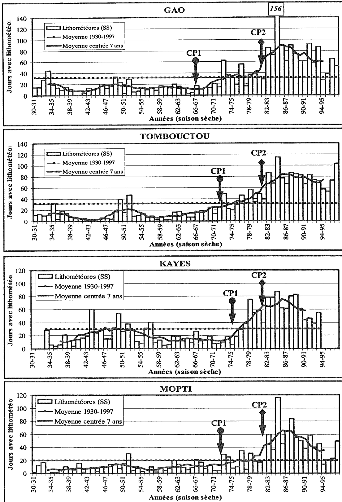
Fig.IV.38 - Evolution des lithomètres en saison sèche (octobre – avril) de 1930-31 à 1997-98 aux stations de Tombouctou, Gao, Mopti et Kayes. La courbe moyenne (pointillés) détermine la période utilisée pour chaque station. CP1 et CP2 indiquent les deux ruptures de tendances.
