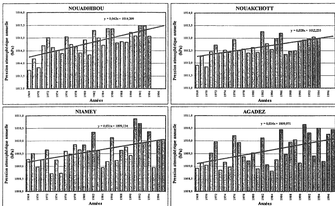
Fig.V.20 - Evolution de la pression atmosphérique (hPa) moyenne annuelle (mai à avril) en Mauritanie (Nouadhibou et Nouakchott: 1968-1994) et au Niger (Niamey et Agadez: 1968-1997).
