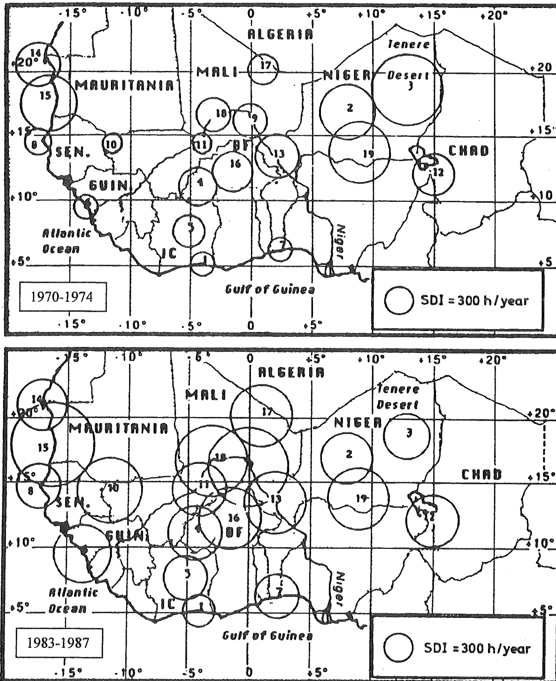
Figure IV. 14: Représentation du nombre d'heures où la visibilité a été inférieure à 500 dam par brume sèche en Afrique de l'Ouest pour les périodes 1970-1974 et 1983-1987. (d'après N'TCHAYI et al. 1994)
