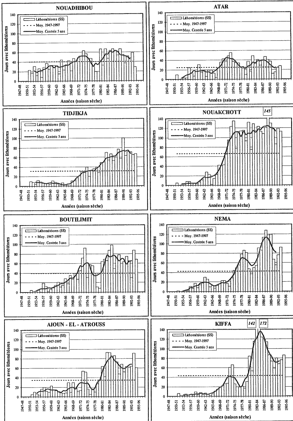
Fig.IV.36 - Evolution du nombre de jours affectés par les lithométéores en saison sèche (octobre – avril) en Mauritanie de 1951-52 à 1994-95. La moyenne détermine la période utilisée pour chaque station.
