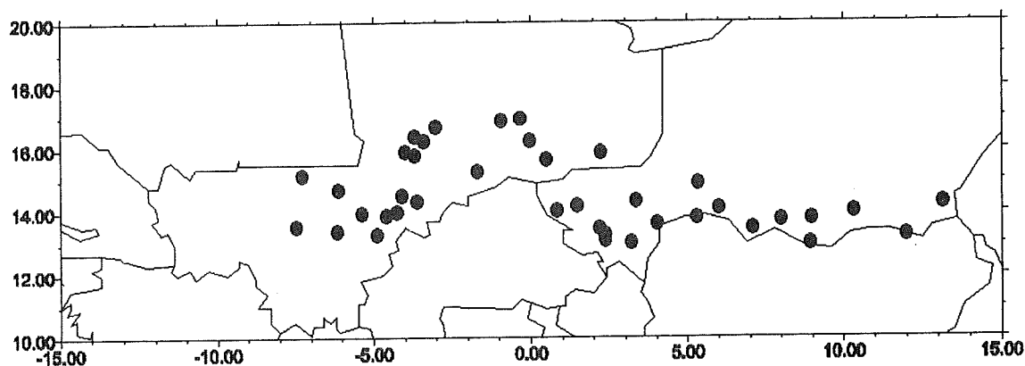
Fig.III.3 - Localisation de stations utilisées pour l'analyse régionale des précipitations. Location of the stations used for the rainfall regional analysis.
