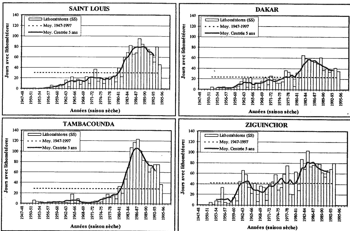
Fig.IV.37 - Evolution du nombre de jours affectés par les lithométéores en saison sèche (octobre – avril) au Sénégal de 1951-52 à 1994-95. La moyenne détermine la période utilisée pour chaque station.
