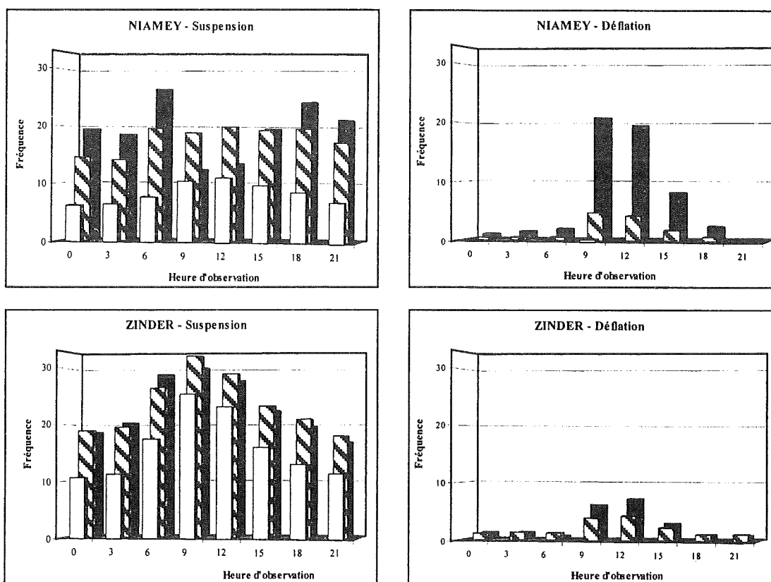
Fig.IV.24 - Fréquence moyenne (%) tri-horaire de la visibilité réduite par les poussières en suspension et les cas de déflation durant la saison sèche (novembre à mars) aux stations de Niamey et Zinder. Comparaison entre les périodes "humide" (1951-1968, blanc), de sécheresse (1969-1986, hachuré), et "actuelle" (1987-1997, noir).
