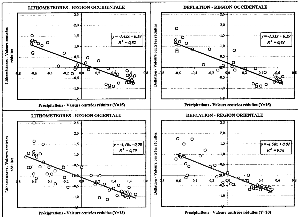
Fig.IV.61 - Relation maximum entre la pluviométrie moyenne régionale et la fréquence régionale des lithométéores et des cas de déflation. Les paramètres sont traduits en valeurs centrées réduites suivant la méthode de LAMB (1982).
