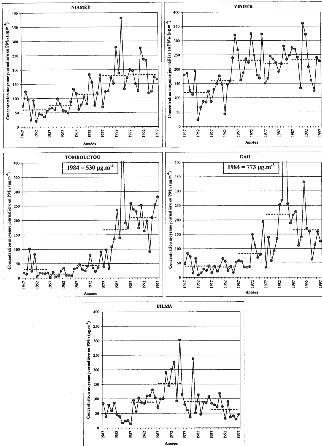
Fig.IV.74 - Concentration journalière moyenne ( \mu\text{g.m}^{-3} ) en particules solides < 10 \mu\text{m} ( \text{PM}_{10} ) dérivée de la l'équation de D'ALMEIDA (1986) en cinq stations synoptiques durant la saison sèche (novembre à mars).
