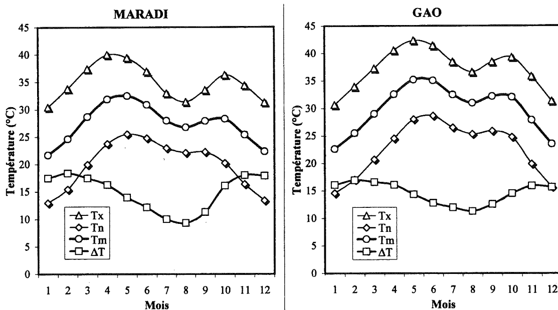
Fig.VI.1 - Répartition mensuelle des températures maximales (Tx), minimales (Tn), moyennes (Tm) et de l'amplitude thermique diurne ( \Delta T ) aux stations de Maradi (Sahel méridional) et de Gao (Sahel septentrional). Données de la période 1951-1997.
