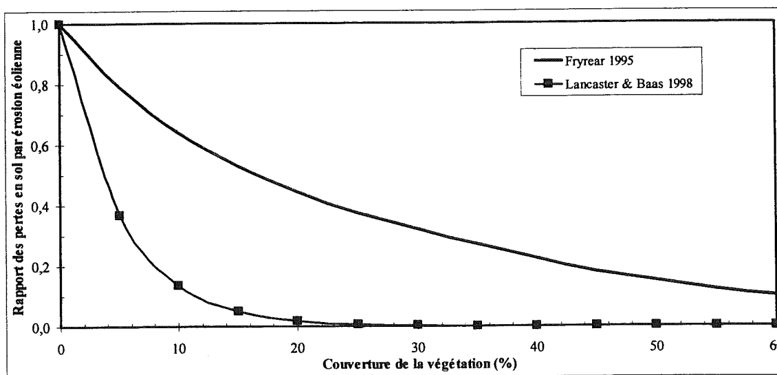
Fig.IV.62 - Relation entre le rapport des pertes en sol (pertes en sol suivant le pourcentage de couverture divisé par les pertes en sol pour une couverture nulle) et pourcentage de la couverture du sol (d'après FRYREAR 1995 et LANCASTER & BAAS 1998)
