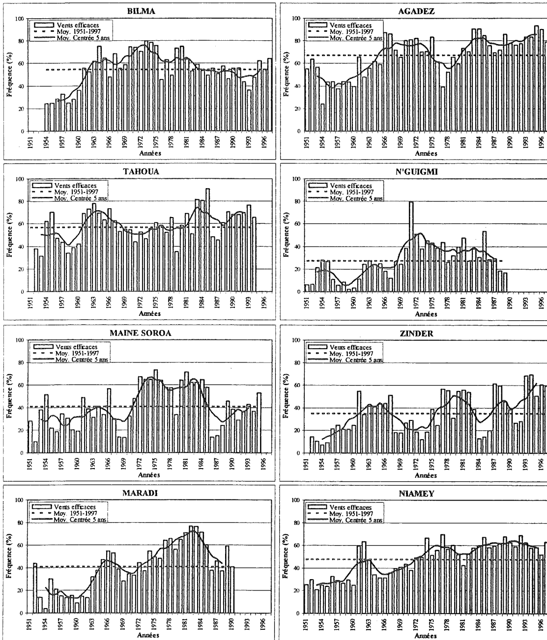
Fig.V.18 - Evolution annuelle de la fréquence des vents efficaces [V_{10(6)}] au Niger de 1951 à 1997. Yearly evolution of the threshold wind speed frequency [V_{10(6)}] in Niger from 1951 to 1997.
