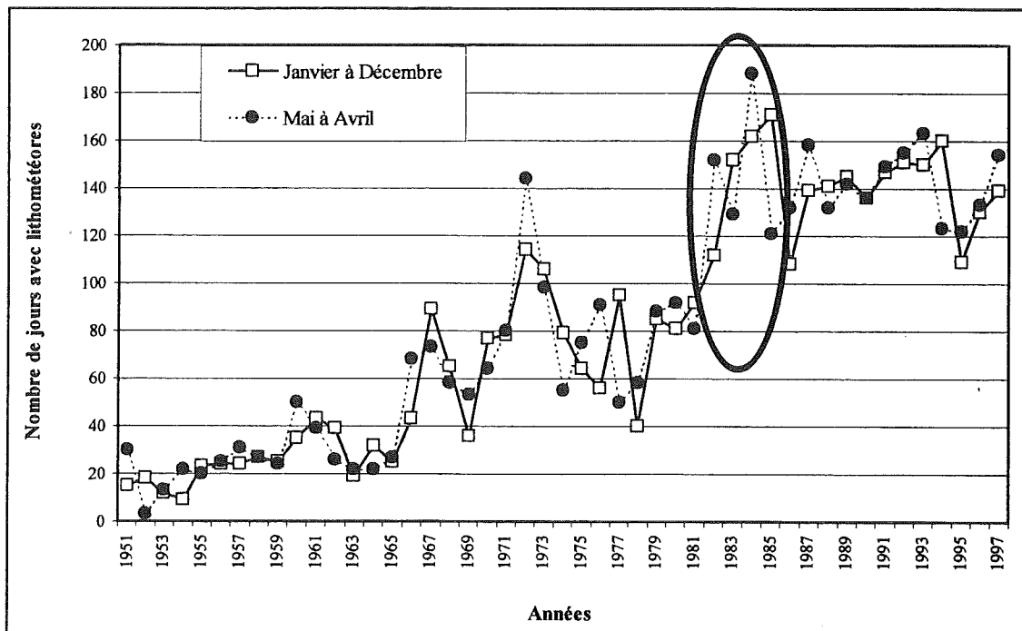
Fig.IV.31 - Evolution annuelle du nombre de jours avec lithométéores à Niamey de 1951 à 1997. Comparaison entre les résultats obtenus entre une année calendrier (janvier à décembre) et une année calquée sur les saisons (mai à avril). Le cercle met en évidence les années 1982 à 1985.
