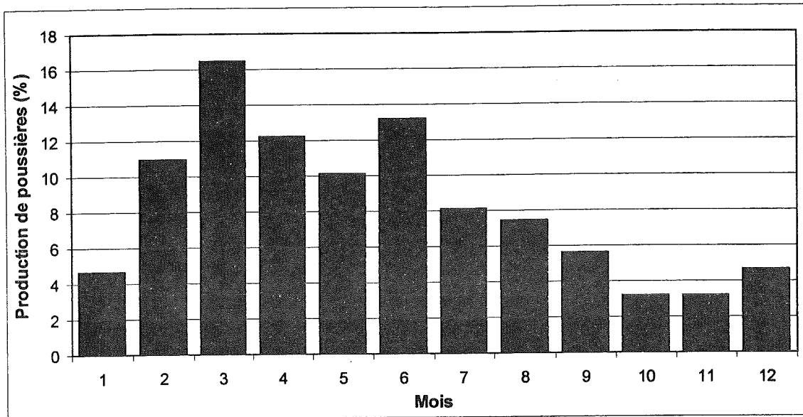
Fig.IV.70 - Répartition mensuelle (en %) de la production de poussière en Afrique sahélienne (d'après D'ALMEIDA 1986).
