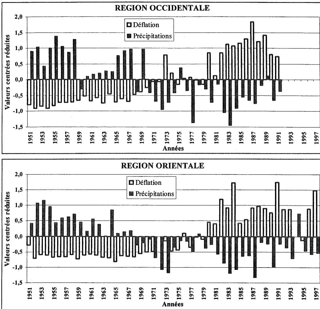
Fig.IV.60 - Evolution des précipitations et des cas de déflation en saison sèche (octobre – avril) de 1951 à 1997 dans les régions occidentale et orientale de la zone d'étude. Les deux paramètres sont traduits en valeurs centrées réduites suivant la méthode de LAMB (1982).
