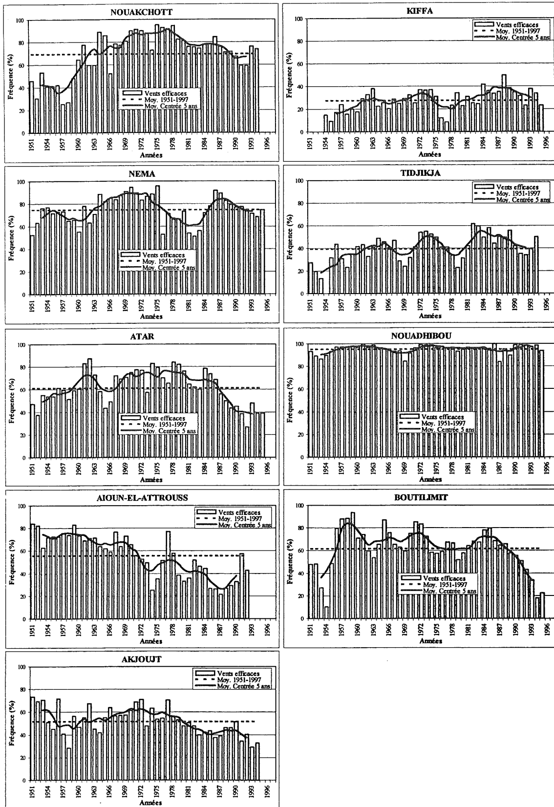
Fig.V.17 - Evolution annuelle de la fréquence des vents efficaces [V_{10(6)}] en Mauritanie de 1951 à 1995. Yearly evolution of the threshold wind speed frequency [V_{10(6)}] in Mauritania from 1951 to 1995.
