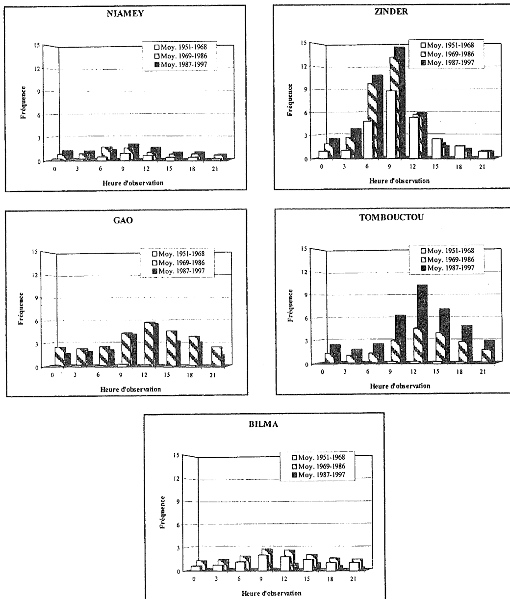
Fig.IV.23 - Fréquence moyenne (%) trihoraire de la visibilité réduite par les lithométéores à moins de 100 dam durant la saison sèche (novembre à mars). Comparaison entre les périodes "humides" (1951-1968), de sécheresse (1969-1986) et
