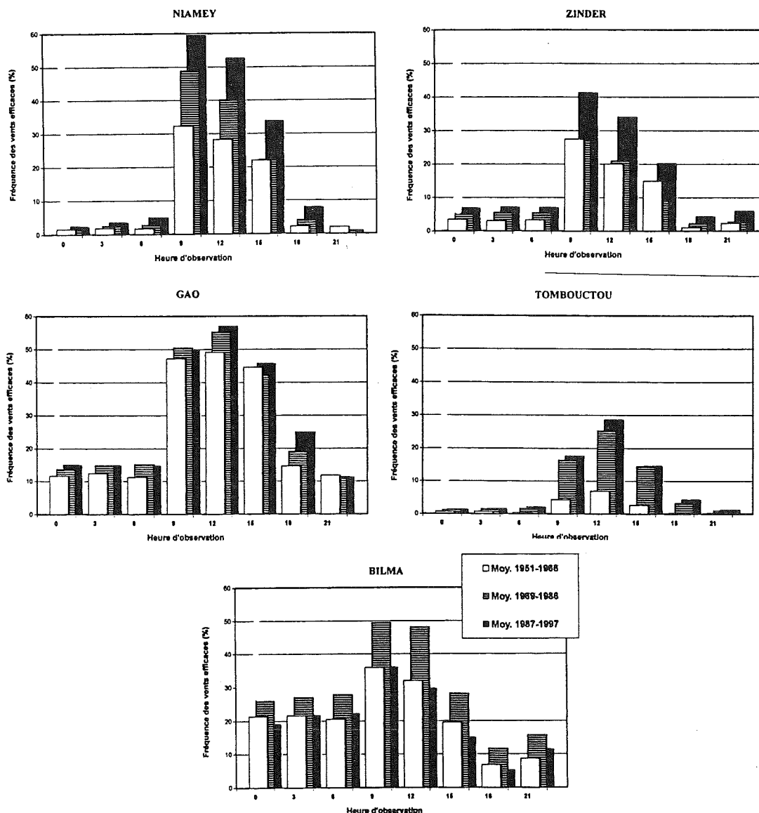
Fig.V.13 - Fréquence moyenne (%) tri-horaire des vents efficaces [V_{10(6)}] durant la saison sèche (novembre à mars). Comparaison entre les périodes "humide" (1951-1968), de sécheresse (1969-1986) et "actuelle" (1987-1997).
