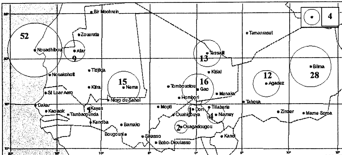
Fig.V.7 - Importance de la déflation potentielle dans onze stations en Afrique de l'Ouest. La taille des cercles est proportionnelle à la valeur E (Eq. V. 3) qui est reportée en valeur chiffrée sur le cercle (d'après CLARK et al. 1997, modifiée).
