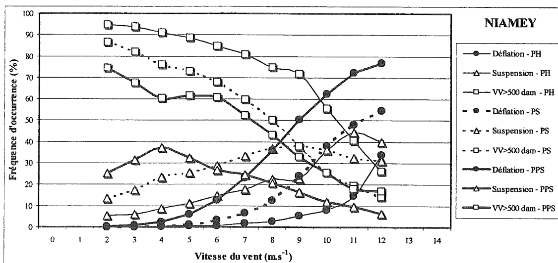
Fig.V.24 - Evolution de la fréquence d'observation des jours sans lithométéore, avec poussière en suspension et avec déflation en fonction de la vitesse du vent ( m s^{-1} ) à Niamey. Comparaison entre les périodes "humide" (1951-1968), de sécheresse (1969-1986) et "actuelle" (1987-1997).
