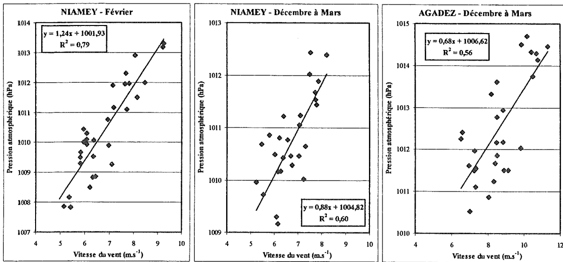
Fig.V.22 - Relation entre la pression atmosphérique (hPa) et la vitesse moyenne du vent en février à Niamey et au cœur de la saison sèche (décembre à mars) à Niamey et à Agadez (1968-1997).
