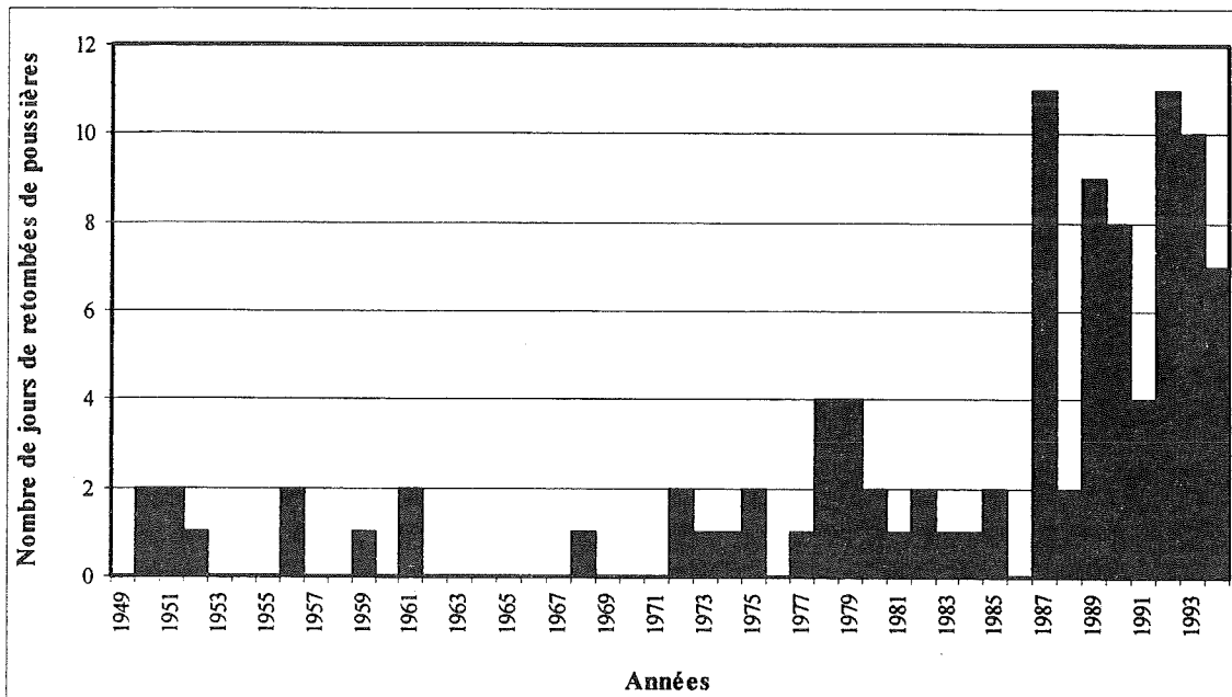
Fig.IV.2 - Evolution du nombre annuel de jours ayant enregistré des retombées de poussières sahariennes à l'observatoire d'Elche (Espagne) de 1949 à 1994 (d'après SALA et al. , 1996).
