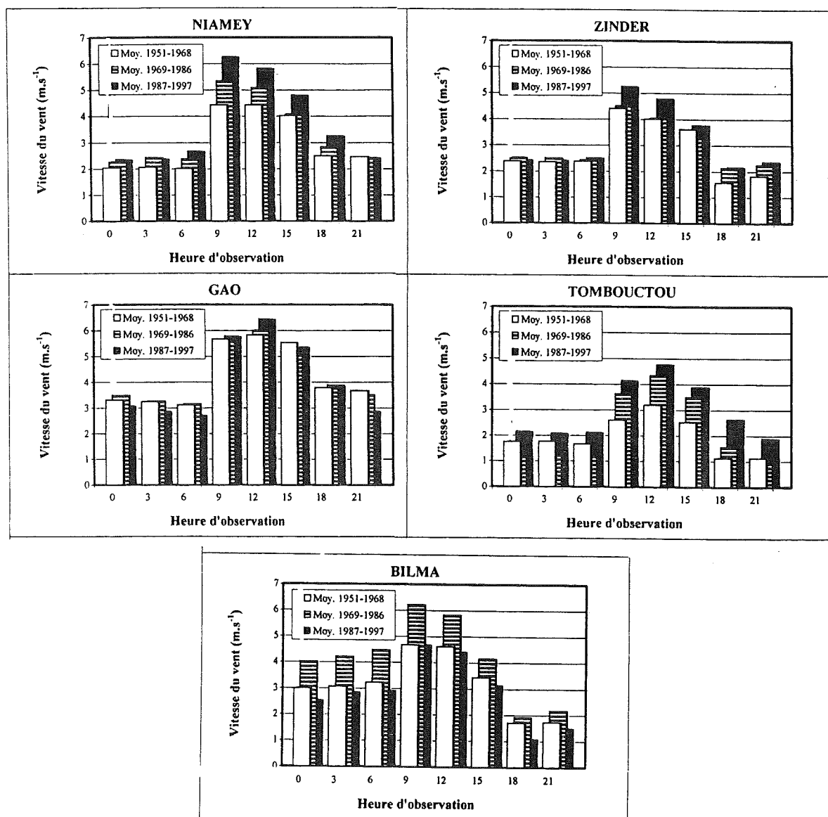
Fig.V.11 - Vitesse moyenne tri-horaire du vent durant la saison sèche (novembre à mars). Comparaison entre les périodes "humide" (1951-1968), de sécheresse et "actuelle" (1987-1997).
