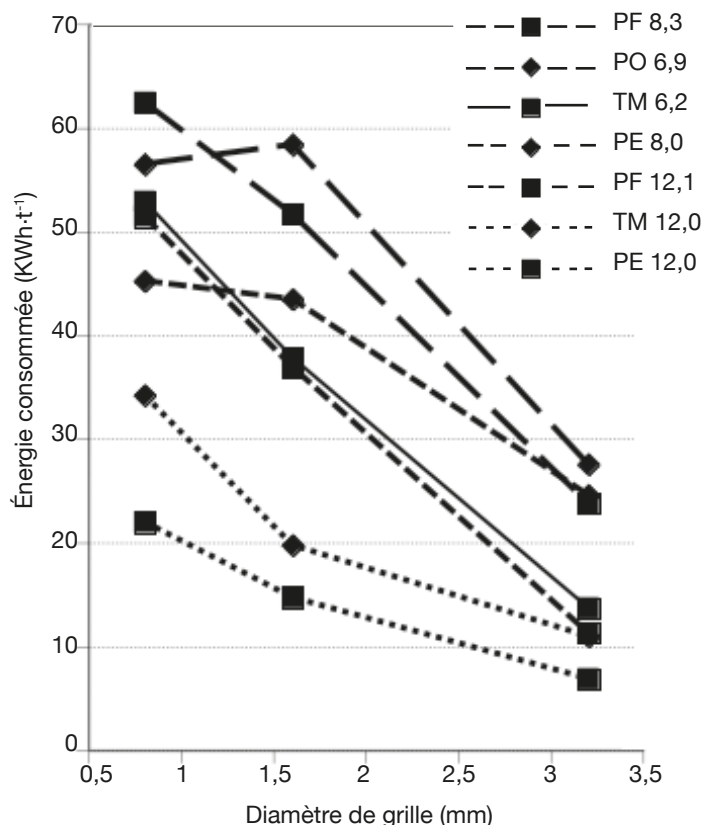
Figure 1. Consommation énergétique nécessaire au broyage de différentes biomasses, à deux niveaux d'humidité et trois diamètre de grille de broyeur (données d'après Mani et al., 2004) — Energy consumption needed for biomass milling, at two moisture content levels, for three hammermill grid diameter (data from Mani et al., 2004).
