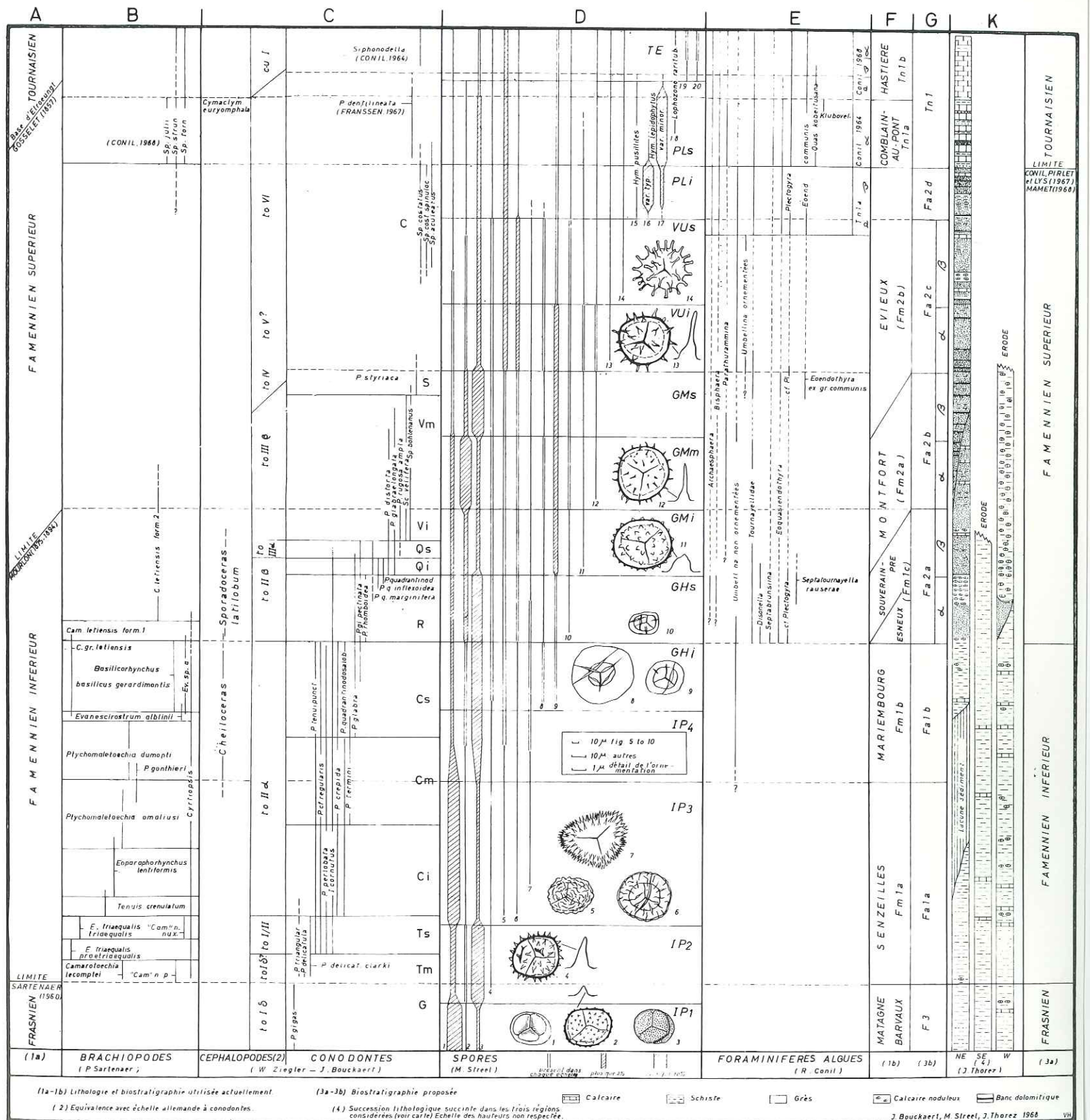
Biostratigraphie et lithostratigraphie du Famennien dans le synclinorium de Dinant (Belgique).
