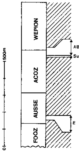
Fig. 98. - Position des biozones par rapport aux différentes formations dans la coupe d'Acoz.
