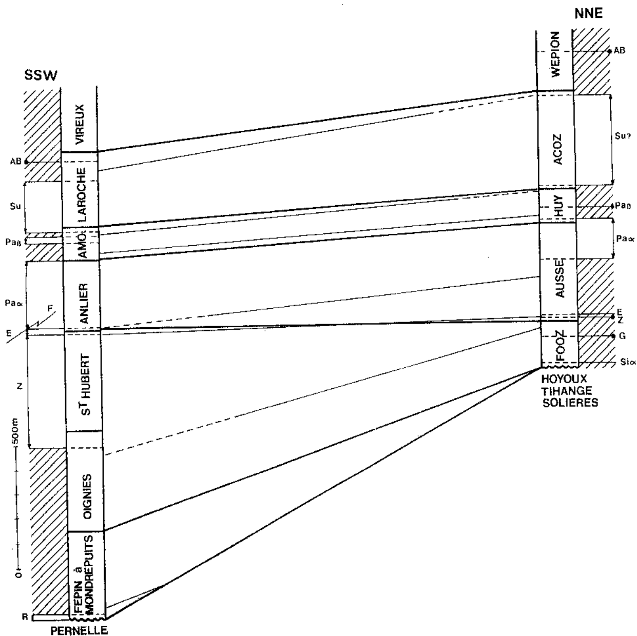
Fig. 125. -- Corrélations biostratigraphiques et lithostratigraphiques entre Pernelle et Hoyoux + Tihange + Solières. Section n° 9. Voir légende fig. 119.
