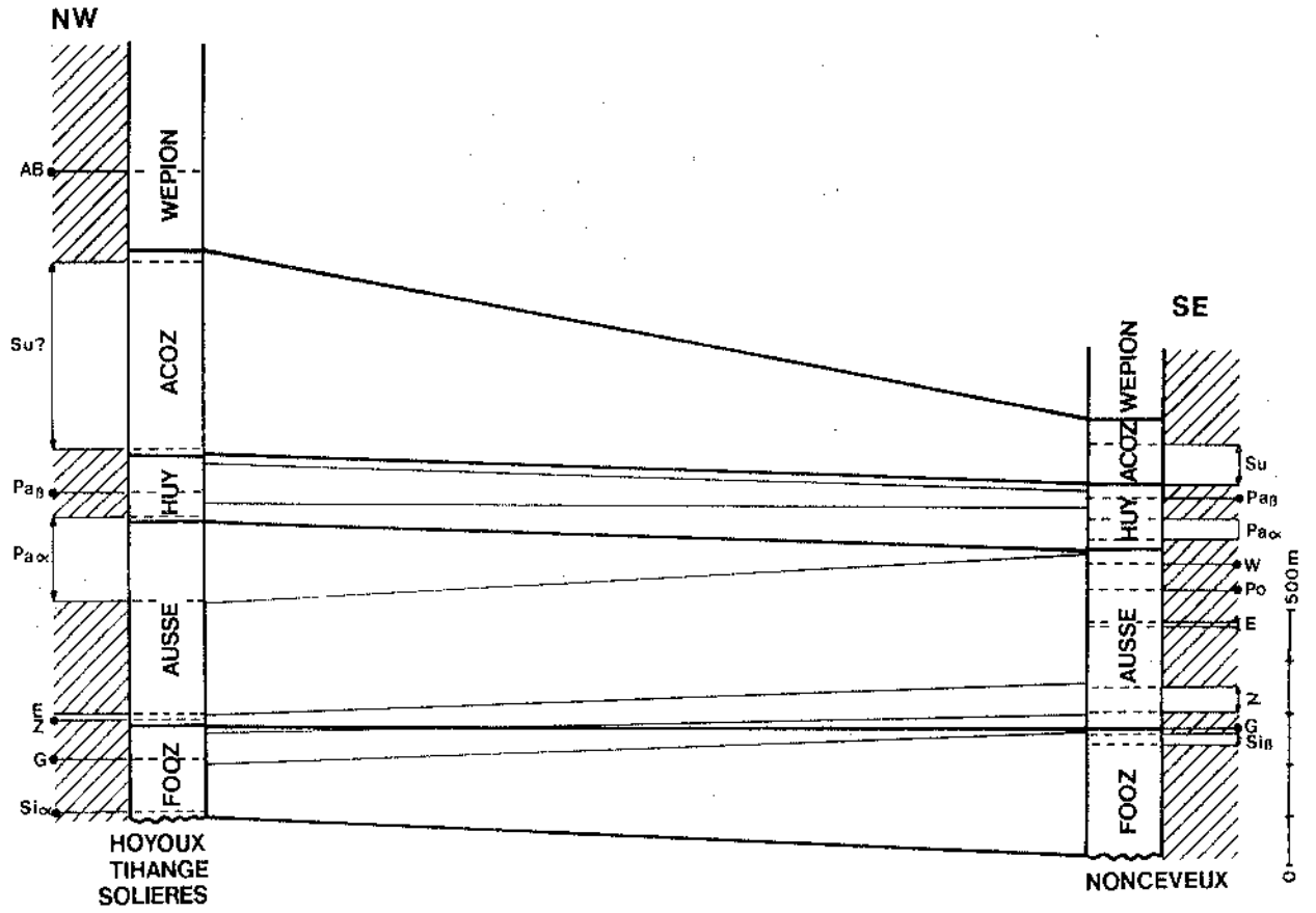
Fig. 121. — Corrélations biostratigraphiques et lithostratigraphiques entre Hoyoux + Tihange + Solières et Nonceveux. Section n° 3. Voir légende fig. 119.
