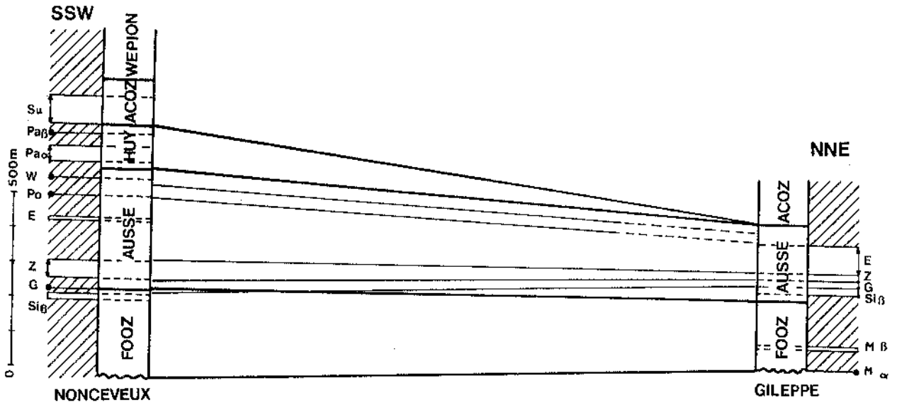
Fig. 123. — Corrélations biostratigraphiques et lithostratigraphiques entre Nonceveux et Gileppe. Section n° 5. Voir légende fig. 119.
