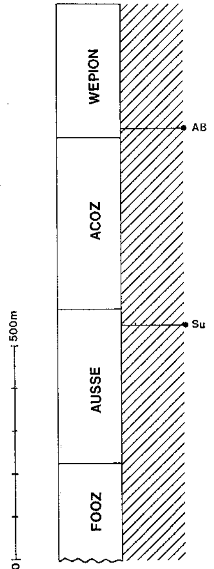
Fig. 96 Position des biozones par rapport aux différentes formations dans la coupe de la vallée du Samson.
