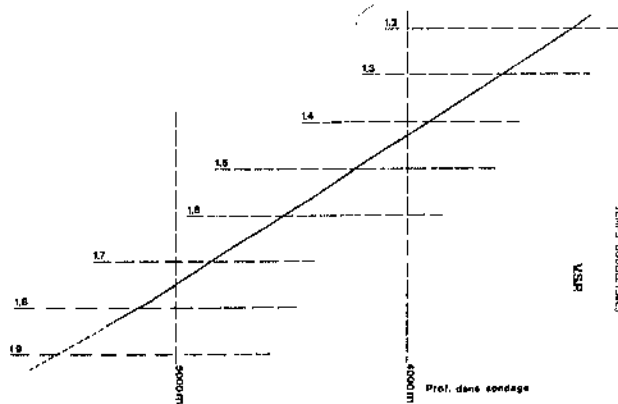
Fig. 113. — Diagramme donnant la correspondance entre temps double et profondeur.
