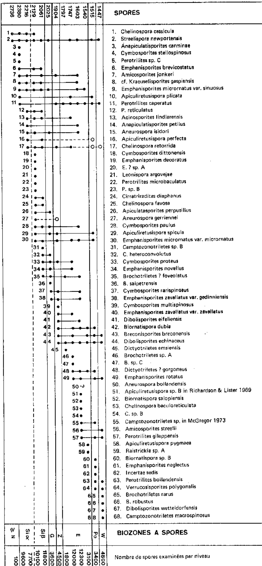
Fig. 102 Distribution stratigraphique des espèces dans le sondage de Bolland (spores). Acriarches voir plus loin.
