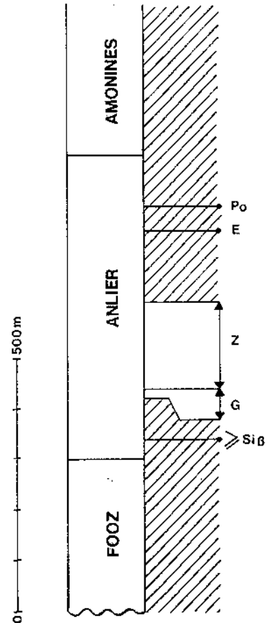
Fig. 90 Position des biozones par rapport aux différentes formations dans la coupe de Manhay.
