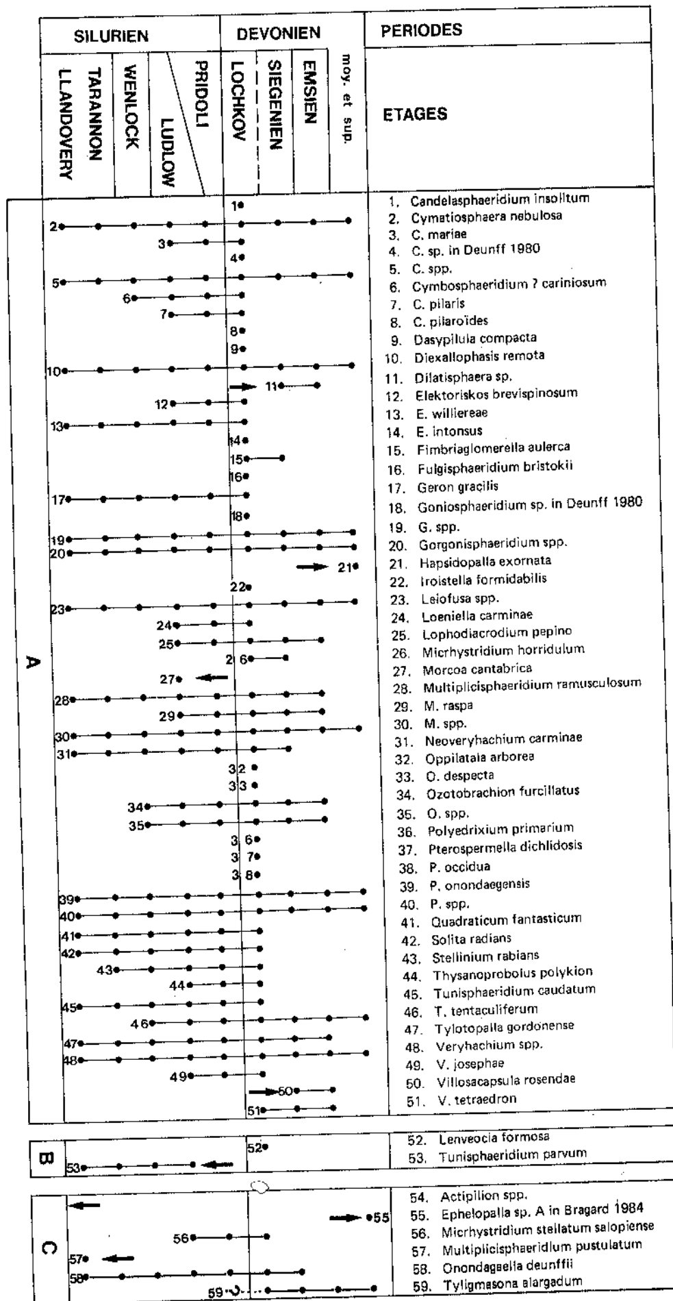
Fig. 214. — Extensions stratigraphiques connues des genres et des espèces d'acritarches déterminés à Saint-Germain-sur-Ay (A) formes propres à Saint-Cénéry (B) et à Chilia (C). Les flèches indiquent les espèces d'âge anormal pour ces niveaux.
