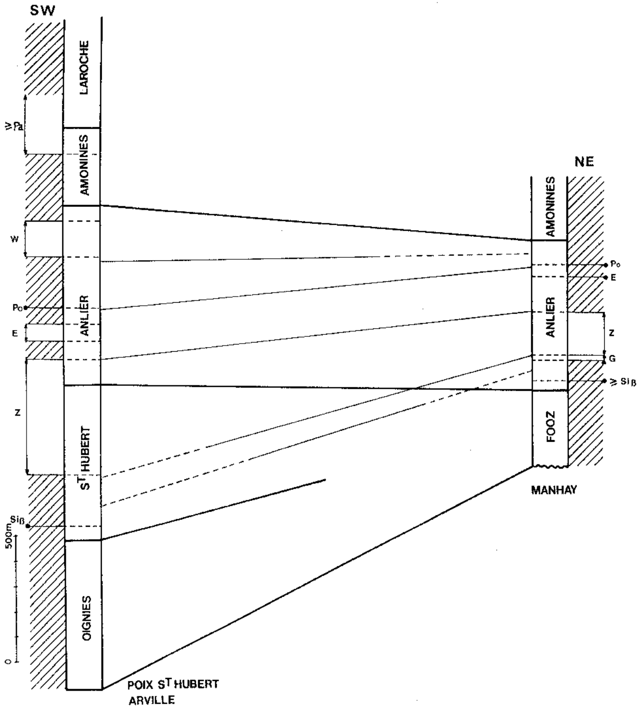
Fig. 120. — Corrélations biostratigraphiques et lithostratigraphiques entre Poix-Saint-Hubert + Arville et Manhay. Section n° 2. Voir légende fig. 119.
