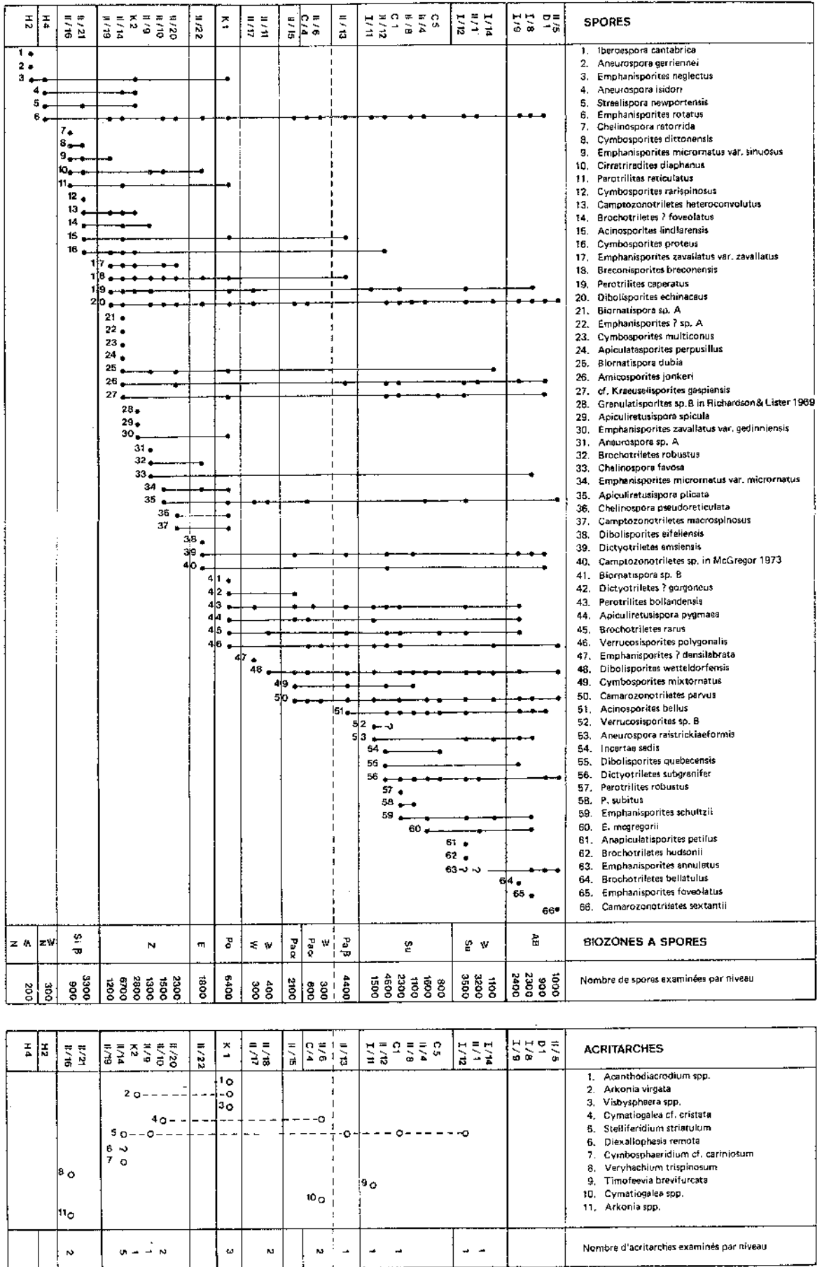
Fig 108. — Distribution stratigraphique des espèces provenant de l'échantillonnage ponctuel réalisé en R.F.A.
