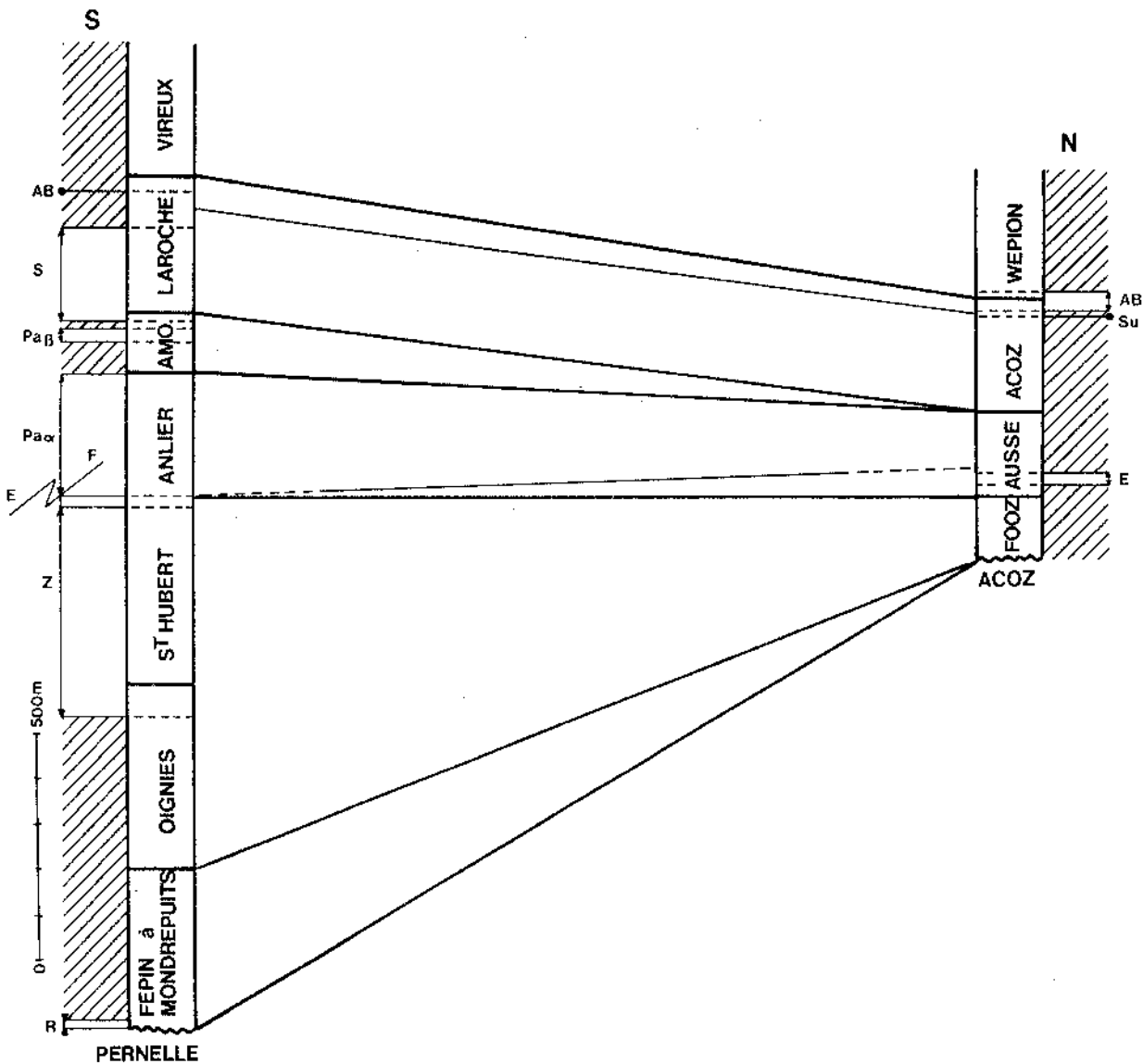
Fig. 130. — Corrélations biostratigraphiques et lithostratigraphiques entre Pernelle et Acoz. Section n° 12. Voir légende fig. 119.
