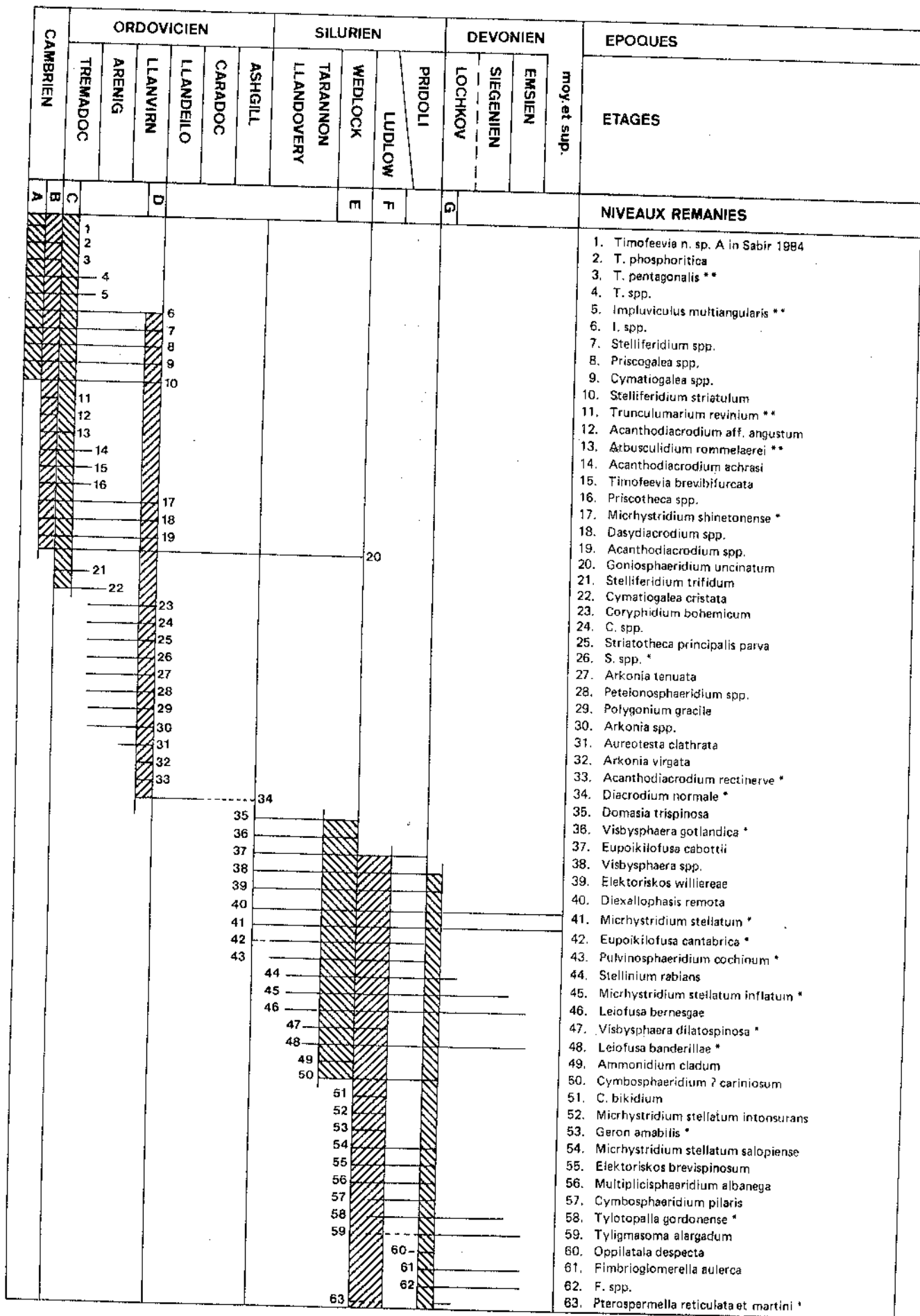
Fig. 219. - Extensions stratigraphiques connues des acritarches non ubiquistes provenant des coupes ardenno-rhénanes.
