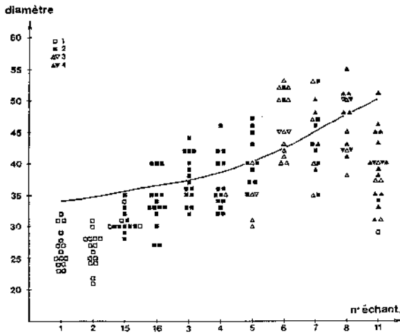
Fig. 71. - Evolution du diamètre des spores en fonction du temps. 1. E. micror-natus var. micror-natus ; 2. E. micror-natus var. sinuosus ; 3. E. zavallatus var. gedinniensis ; 4. E. zavallatus var. zavallatus . Courbe : diamètre moyen de la population totale des spores.
